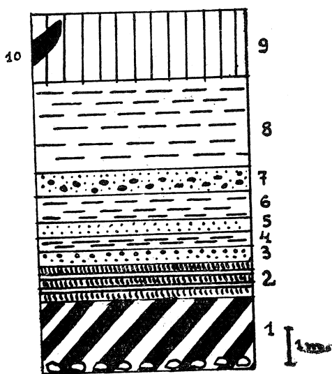
Otoczaki z moreny dennej: 1. Torf. 2. Gytja z wkładkami piasków i żwirków. 3. Otoczaki w piasku. 4. Iły zielone, warstwowane. 5. Piasek warstwowany. 6. Głina zielonkawa warstwowana. 7. Piasek ze żwirkami i otoczkami (— 30 m). 8. Głina żółtawa warstwowana. 9. Gliny lessowate warstwowane. 10. Humus.
