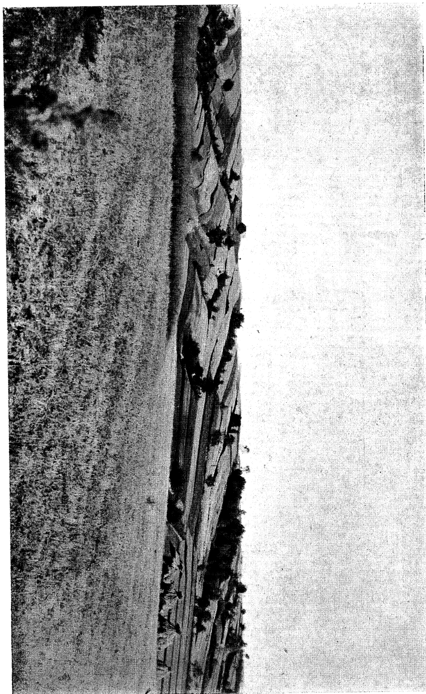
Fig. 8. Wieś Kawęczyn koło Szczepieszyna. Rzeźba wschodniego zbocza (od strony doliny Wieprza) wału Rostocza, w pobliżu kulminacji +332\text{ m} .
