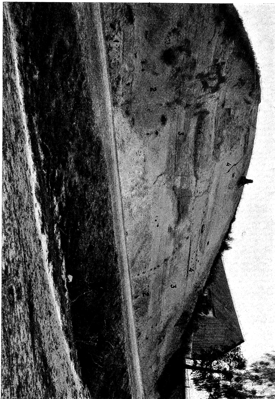
Fig. 6. Dworzyska, zachodnia ściana wykopu. 1 — aluwja piaszczyste, 2 — typowy less subaeralny młodszy górny; 3 — utwór zastoiskowy lessowy; 4 — serja piaszczystych aluwjów rzecznych; w stropie warstwa gleby współczesnej leśnej.
