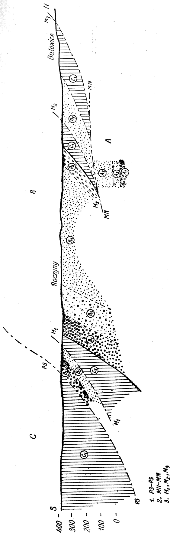
Fig. 5. Miocen autochtoniczny (A): A 1 — zlepience pstre; A 2 — iły z fragmentami fliszowymi (A 1 —A 2 helwet? — torton dolny); A 3 — iły i piaskowce z heterosteginami — podpietro opolskie. Miocen nasunięty (B): B 1 — zlepience pstre; B 2 — zlepience ciemne; B 3 — iły z fragmentami fliszowymi; B 4 — iły ciemne (B 1 —B 4 — helwet? — torton dolny); B 5 — podpietro opolskie. Jednostka podślaska (C): C 1 — ciemne łupki z syderytami, pstre margle (senon-paleogen).
