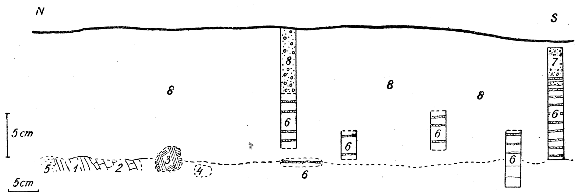
Fig. 3. Przekrój w potoku Roczynka E (na W od Andrychowa): 1 — ciemne ropy (—HCl); 2 — margle zielone; 3 — łupki menilitowe z wkładkami piaskowców glaukonitowych (1—3 eocen podśląski); 4 popielate ropy +HCl (?); 5 — ciemne ropy, torton dolny; 6 — ropy zlepniowate z wkładkami piasków, torton środkowy; 7 — żwiry, pleistocen; 8 — osypisko.
