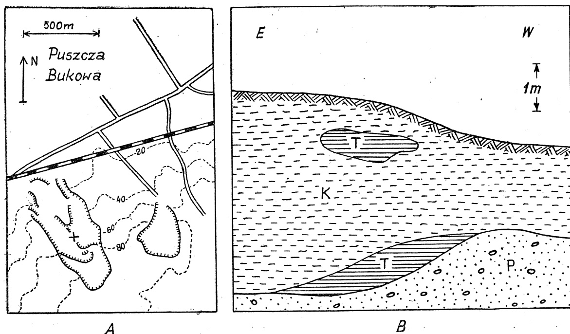
Fig. 1. Odsłonięcie w Puszczy Bukowej. A — Plan sytuacyjny odsłonięcia, Krzyżkiem oznaczono miejsce odsłonięcia; B — Profil odsłonięcia; P — piaski plejstoceńskie; K — margle kredowe; T — utwór ilasty (Quetschbreccie)
