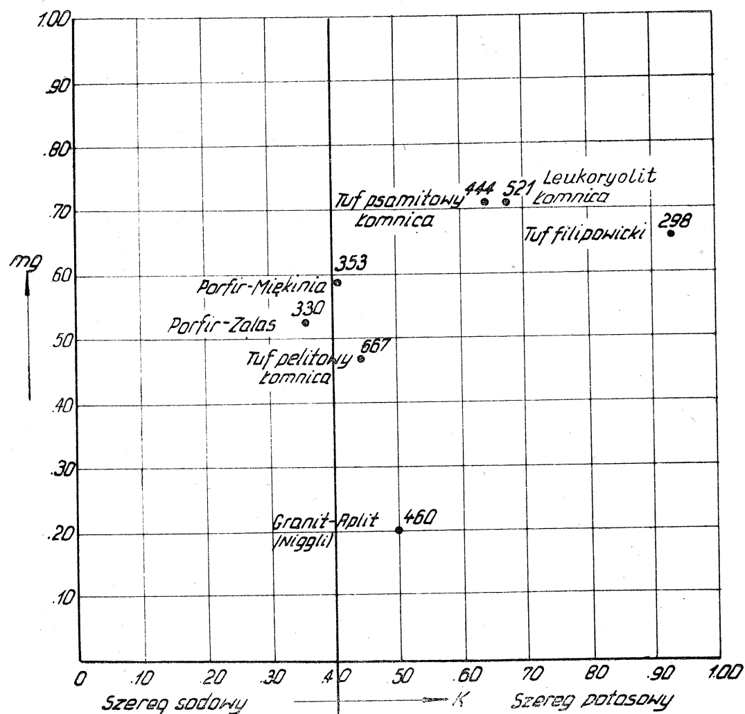
Fig. 3. Diagram K-Mg według Nigglego; cyfry odpowiadają wartościom parametrów si
