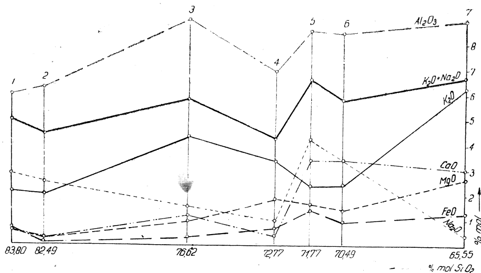
Fig. 2. Diagram wariacyjny według Osanna. 1 — tuf porfirowy pelitowy; 2 — kuleciste agregaty tufu pelitowego; 3 — skała porfirowa z Łomnicy (K-ryolit); 4 — tuf porfirowy psamitowy; 5 — porfir z Zalas; 6 — porfir z Miękinia; 7 — tuf filipowicki.
