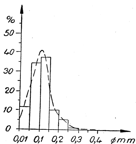
Fig. 3. Typ I. Kwarcyty. Krzywa uziarnienia indywidualna
