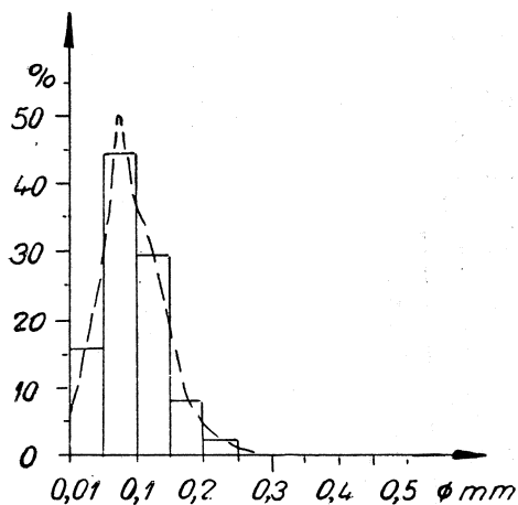
Fig. 8. Typ IV. Piaskowce kruche. Krzywa uziarnienia indywidualna
