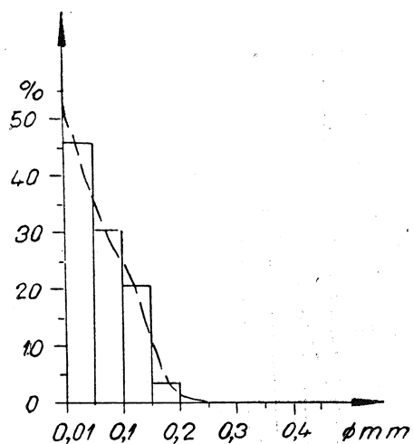
Fig. 6. Typ III. Piaskowce kwarcytowe. Krzywa uziarnienia indywidualna
