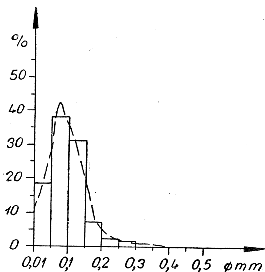
Fig. 2. Typ I. Kwarcyty. Krzywa uziarnienia indywidualna
