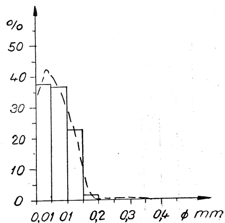
Fig. 7. Typ IV. Piaskowce kruche. Krzywa uziarnienia indywidualna
