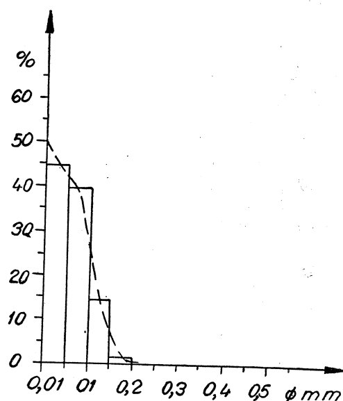
Fig. 5. Typ III. Piaskowce kwarcytowe. Krzywa uziarnienia indywidualna
