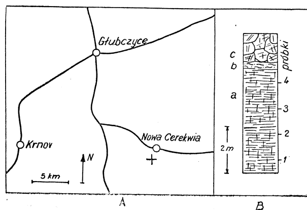
Fig. 1. Odsłonięcie w Nowej Cerekwi. A — mapka sytuacyjna, krzyżkiem oznaczono miejsce odsłonięcia. — B — profil odsłonięcia: a — ily margliste; b — ily piaszczyste; c — bazalt; 1—4 miejsca pobrania próbek
