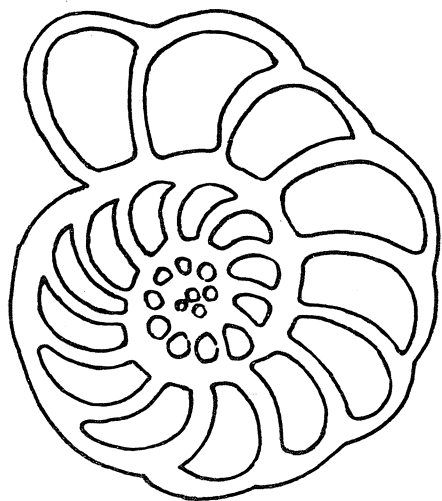
Fig. 3. Cibicides crassiseptatus Łuczowska, forma mikrosferyczna, Mokrzeszów koło Tarnobrzega, górny torton
