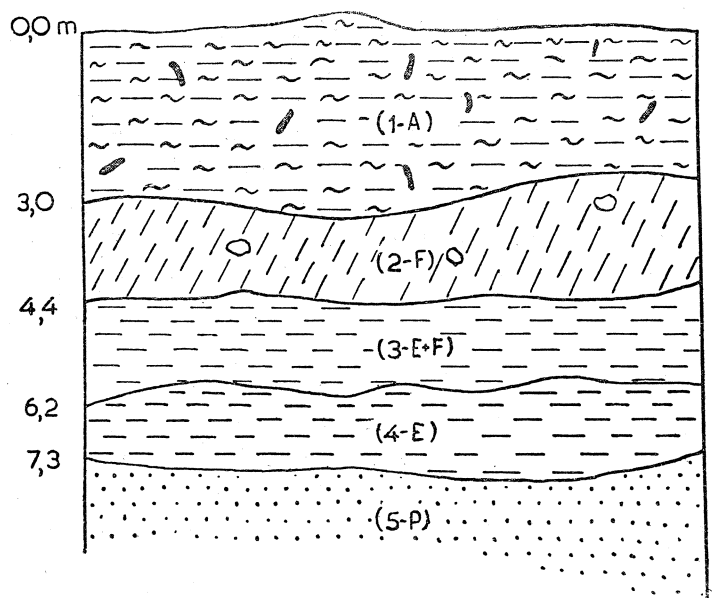
Fig. 3. Profil I z kopalni dolnego poziomu. 1 — ilt mułkowy szarzielony, słabo zwarty ze skorupkami fauny Yoldia (A); 2 — ilt średniotłusty, czekoladowoczerwony, silnie zwarty z pojedynczymi otaczakami skał wapiennych (F); 3 — ilt tłusty szary z wtrąceniami iltu barwy czekoladowej (E + F); 4 — ilt tłusty ciemnoszary, bez fauny, zwarty (E); 5 — piasek drobnoziarnisty barwy szarej (P)
