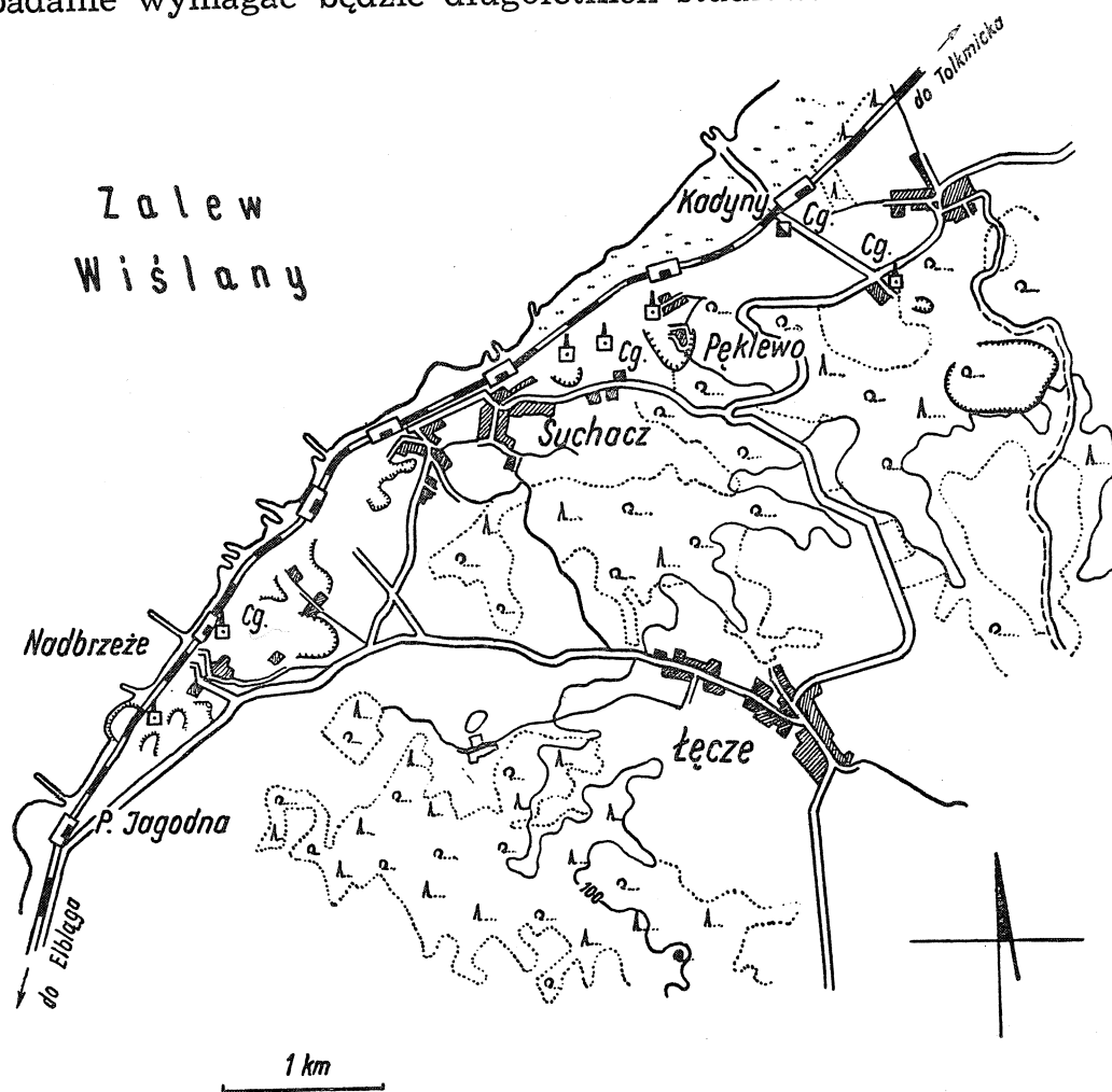
Fig. 1. Mapa odsłoneń iłów elbląskich nad Zalewem Fig. 1. Sketch-map of the clay pits in which the Elbląg clays are exposed
