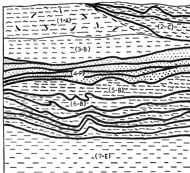
Fig. 4. Obraz zalegania utworów ilastych profilu II. 1 — ił szarzielony mułkowy z resztkami skorup (A); 2 — mułek ilasty z pojedynczą fauną (C); 3 — ił mułkowy szary bez fauny (B); 4 — piasek miękki szary nieco zaburzony z wstawkami mułkowo-ilastymi (P); 5 — ił mułkowy szary z drobnymi przewarstwieniami piasku (B); 6 — ił mułkowy, ciemnoszary z wstawkami mułkowymi, zaburzony (B); 7 — ił tłusty ciemnoszary (E)
