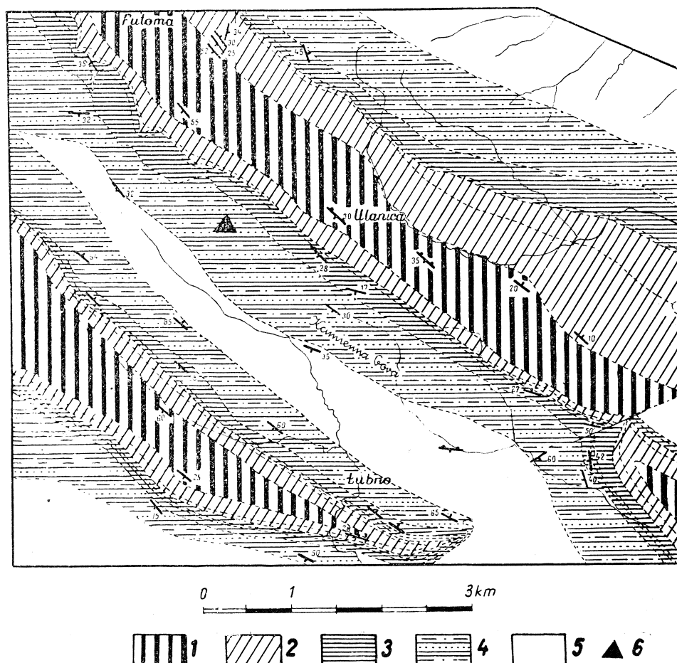
Fig. 2. Mapa geologiczna Łubna (geologia wg J. Wdowiarza): 1 — warstwy inoceramowe, 2 — pstre łupki i warstwy hieroglifowe, 3 — niższa część serii menilitowej, 4 — wyższa część serii menilitowej, 5 — warstwy krośnieńskie, 6 — stanowisko ryb w łupkach jasielskich
