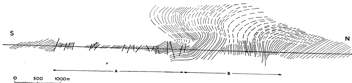
Fig. 3. Fałd leżący w odsłonięciu w dolinie rzeki Kacwińskiej. A strefa uskoków przed czołem fałdu, B strefa fałdu (W. Prokopek 1960)
