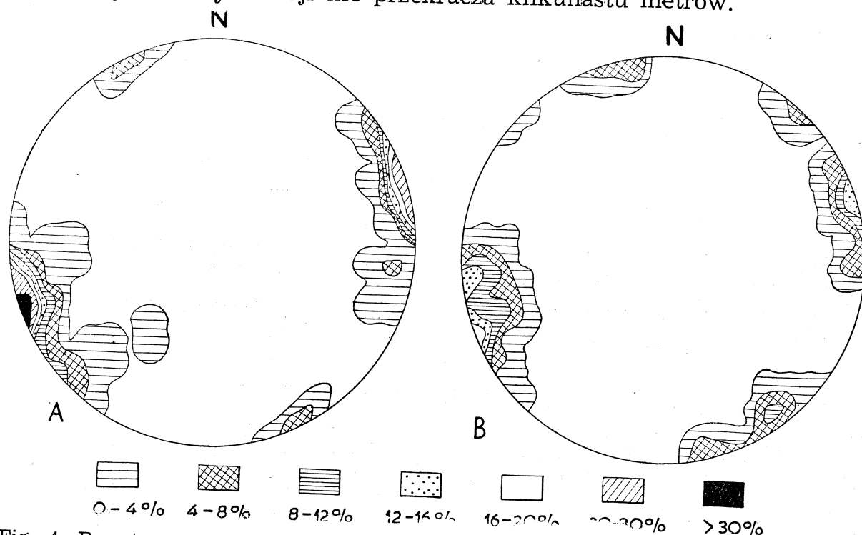
Fig. 4. Przestrzenne ułożenie osi mikroantyklin na obszarze wschodniego Podhala. Naniesiono pomiary 96 antyklin. A dolina Poronca, B obszar Galicowej Grapy i strefy osiowej niecki Podhala (J. Pokorski 1962)
