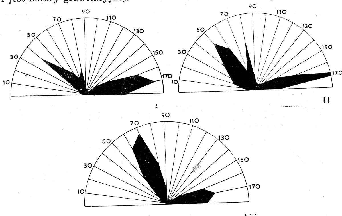
Fig. 5. Diagramy kierunków spękań ciosowych we fliszu podhalańskim. I elewacja Zgorzelisk, II strefa osiowa niecki, III Galicowa Grapa i obszary przyległe (J. Pokorski 1962)
