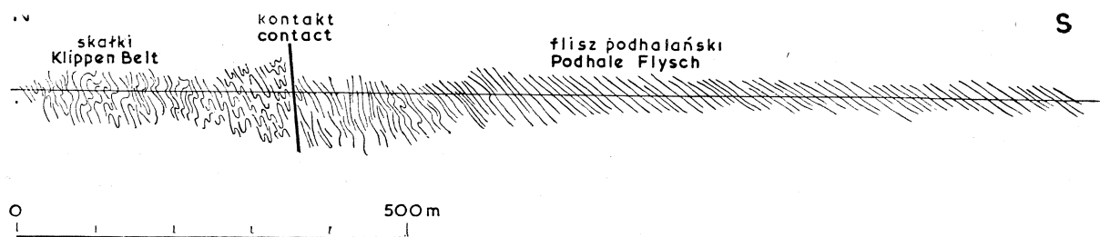
Fig. 1. Strefa kontaktowa fliszu podhalańskiego z pienięskim pasem skałkowym w dolinie Białego Dunajca w Szaflarach
