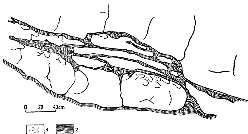
Fig. 7. Fragment osuwiska podmorskiego (warstwa 5). 1 — wapienie; 2 — margle
