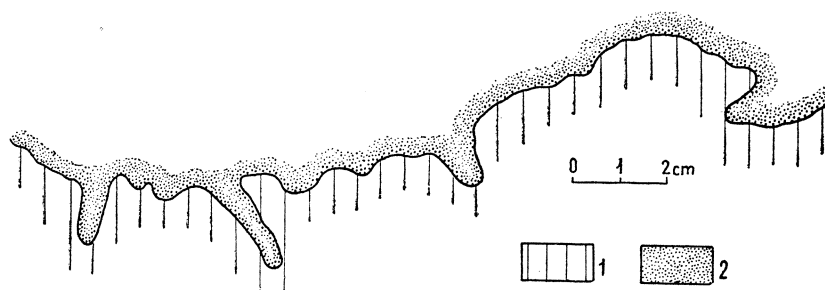
Fig. 6. Powierzchnia rozmycia w spągu ławicy zlepieńca śródformacyjnego (warstwa 6). 1 — wapień z Calcisphaera ; 2 — wapień pseudooolitowy
