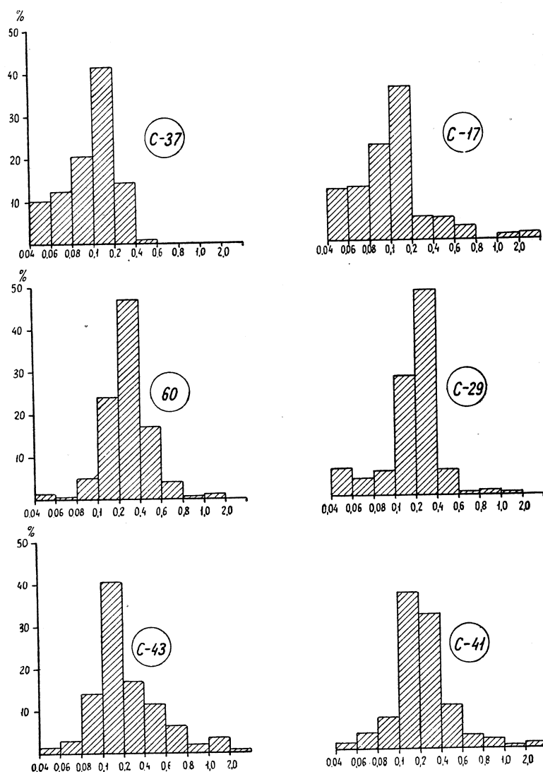
Fig. 3. Skład granulometryczny wapieni pseudoolitowych. Próbki: C-41, C-43 — z warstwy 3; C-29, 60, C-37 — z warstwy 6; C-17 — z warstwy 7
