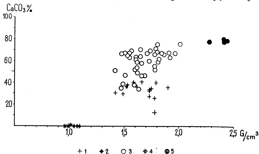
Fig. 7. Zawartość CaCO 3 i ciężar objętościowy skał niższej części dolnego mastrychtu. 1 — gezy wapniste glaukonitowe; 2 — gezy glaukonitowe odwapnione; 3 — opoki, gezy wapniste i margle; 4 — gezy odwapnione; 5 — wapienie piaszczyste
