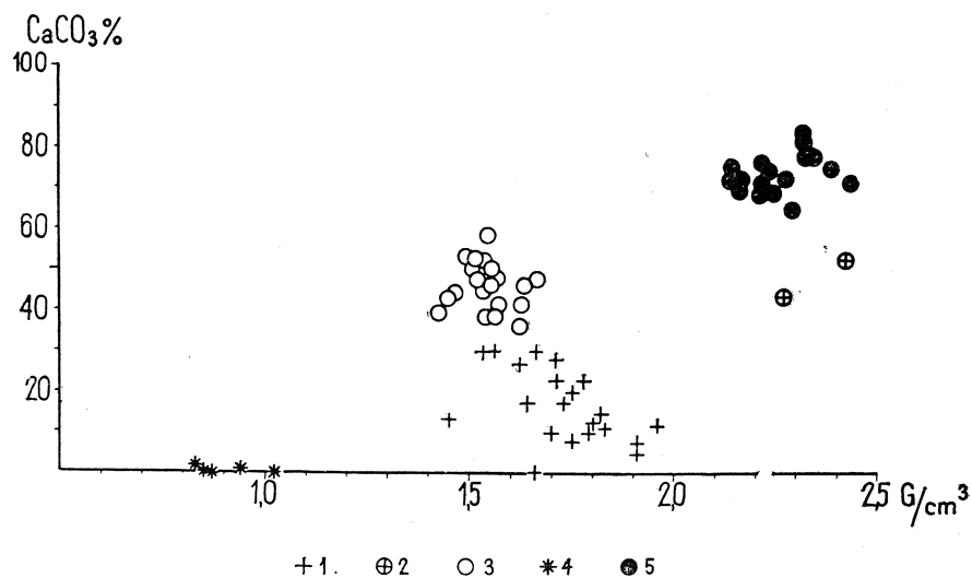
Fig. 8. Zawartość \text{CaCO}_3 i ciężar objętościowy skał wyższej części dolnego mastrychtu. 1 — piaskowce, gezy wapniste, margle piaszczyste ze spągowej części serii; 2 — piaskowce silnie wapniste; 3 — gezy wapniste i opoki; 4 — gezy odwapnione; 5 — wapienie
