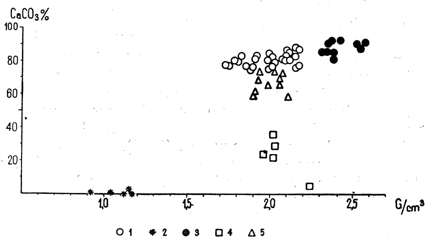
Fig. 4. Zawartość \text{CaCO}_3 i ciężar objętościowy skał wyższej części dolnego kampanu. 1. wapienie margliste i opoki; 2 — opoki odwapnione; 3 — wapienie twardego dna; 4 — czerty; 5 — margle
