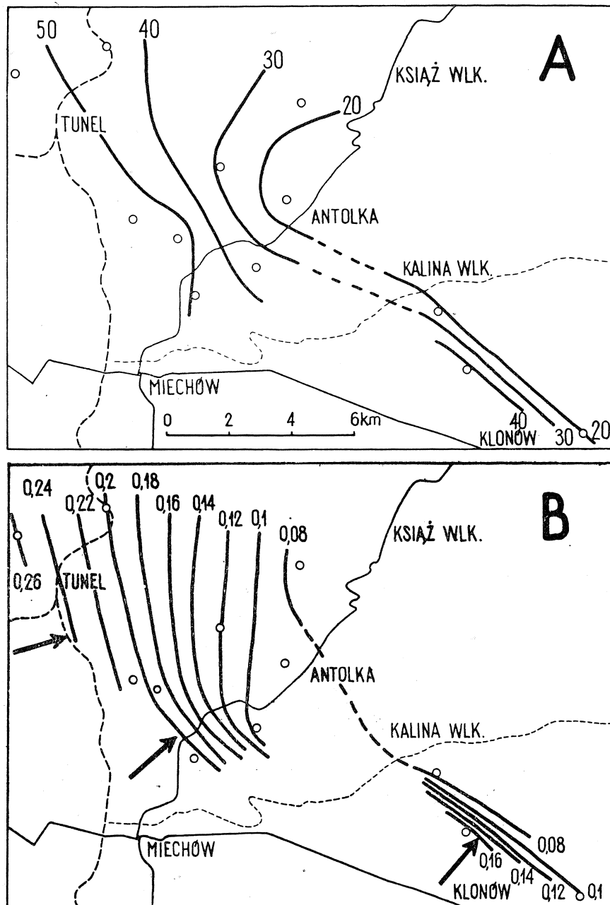
Fig. 11. Zmienność osadów i kierunki transportu w spągowej części trzeciego cyklu sedimentacyjnego. A — Izolinie procentowej zawartości składników detrycznych;
