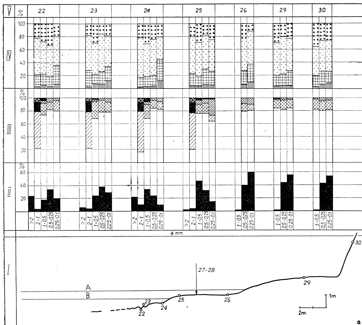
Fig. 3. I — Ustka profile 3; II — skład mechaniczny; III — skład mineralno-petrograficzny; IV — obtoczenie ziarn kwarcu; V — próbka nr; Objaśnienie sygnatur jak na fig. 1.
