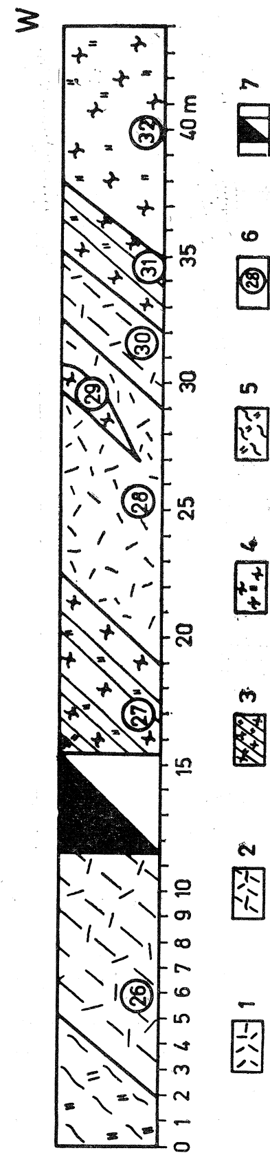
Fig. 5. Rozdroże Izerskie. Profil poprzeczny żyły kwarcowej na linii sztolni II (profil ociosów południowych przecinki nr 1 i 2). 1 — kwarc żyłny; 2 — kwarc o teksturze kierunkowej z relikdami skały pierwotnej; 3 — gnejs z grubymi laminami i wkładkami kwarcu; 4 — gnejs skrzemionkowany; 5 — łupek kwarcowo-łyszczkowy; 6 — lokalizacja i numer pobranej próby; 7 — sztolnia. Fig. 5. Rozdroże Izerskie. Transversal profile of the quartz vein — adit II. Profile of the cross-cuts No. 1 and No. 2, south faces: 1 — vein quartz; 2 — quartz with directional structure and relictst of the primary rock; 3 — gneiss with thick laminae and intercalations of quartz; 4 — silicified gneiss; 5 — quartz-mica schist; 6 — localization of samples; 7 — adit
