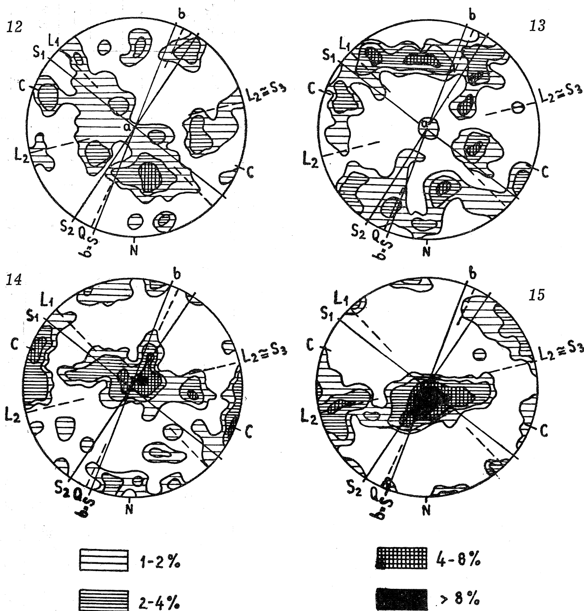
Fig. 3 C. Rozdroże Izerskie. Diagramy konturowe dla 100 osi optycznych kwarcu w próbkach 12, 13, 14, 15; Q, L_1 , L_2 — spekanie; S, S_1 , S_2 , S_3 — płaszczyzny ślizgu; a, b, c — osie teksturalne
