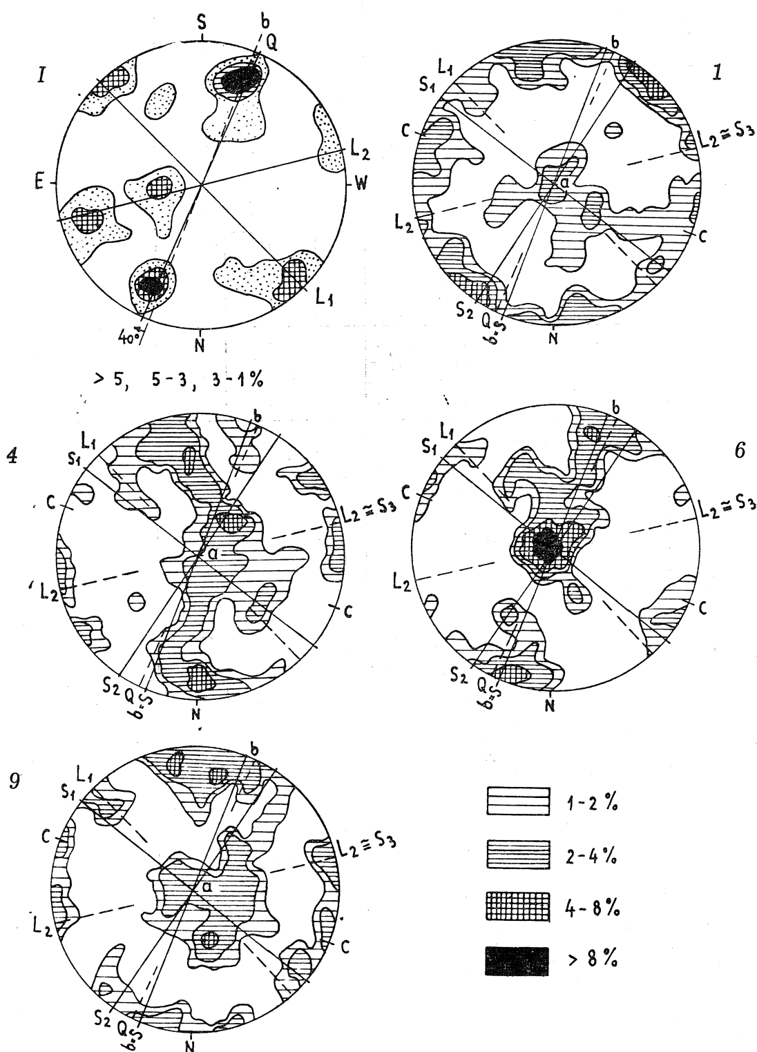
Fig. 2 D. Rozdroże Izerskie. I — stereograficzny wykres spękań w żyłę kwarcowej; Q — spękania podłużne; L 1 i L 2 — spękania poprzeczne; b — rozciągłość żyły; pr. 1, 4, 6, 9 — diagramy konturowe dla 100 osi optycznych kwarcu w próbach nr 1, 4, 6, 9 (patrz fig. 2 A), rzut na dolną półkulę; Q, L 1 , L 2 — spękania; S, S 1 , S 2 , S 3 — płaszczyzny ślizgu; a, b, c — osie teksturalne
