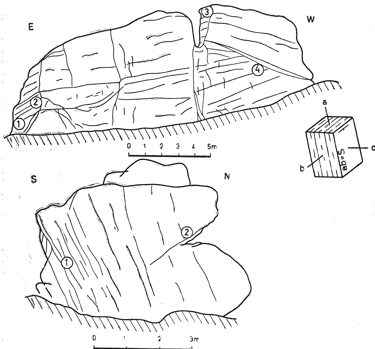
Fig. 7. Pasiecznik, profil skałki kwarcowej na górze Bojanka: A — orientacja przestrzenna elementów teksturalnych pobranych prób
