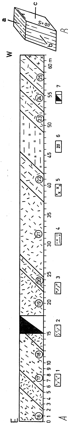
Fig. 4 A, B. Rozdroże Izerskie. A — profil poprzeczny żyły kwarcowej na linii sztolni I, wzdłuż przecinki nr 1 i 2 (ociosy południowe); 1 — kwarc żylny; 2 — kwarc o teksturze kierunkowej (z relikтами skały pierwotnej); 3 — łupek kwarcowo łyszczykowy; 4 — skała kwarcowa z kavernami wypełnionymi substancją ilastą i szczotkami kwarcowymi; 5 — gnejs skrzemionkowany; 6 — lokalizacja i numer pobranej próby; 7 — sztolnia: B — orientacja przestrzenna elementów teksturalnych pobranych próbek
