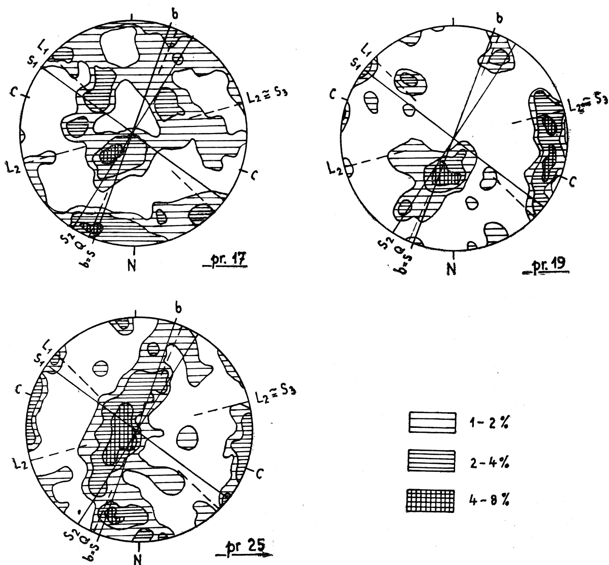
Fig. 4 C. Rozdroże Izerskie. Diagramy konturowe dla 100 osi optycznych kwarcu w próbach 17, 19, 25 (patrz fig. 4 A), symbole jak na fig. 3 C
