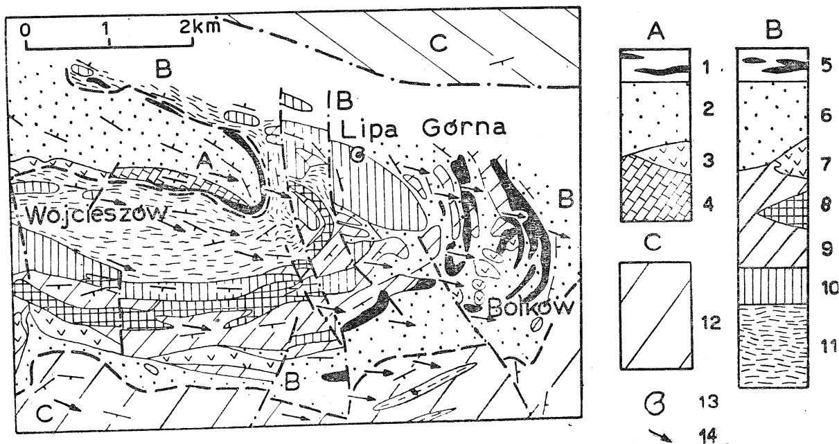
Fig. 1. Szkicowa mapa geologiczna okolicy Lipy Górnej (według H. Teisseyra 1963). A — jednostka Świerzawy: 1 — lidyty i łupki — sylur, 2 — szare łupki — ordowik, 3 — keratofiry-ordowik, kamb, 4 — łupki zielencowe — kamb wyższy. B — jednostka Bolkowa: 5 — lidyty i łupki — sylur, 6 — szare łupki — ordowik, 7 — keratofiry — ordowik, kamb, 8 — porfiry — kamb wyższy, 9 — łupki zielencowe — kamb wyższy, 10 — wapień wojcieszowskie — kamb dolny (i częściowo środkowy?), 11 — warstwy (łupki) radzimowickie — eokamb. C — jednostka Dobromierza: 12 — łupki zielencowe z wkładkami łupków chlorytowych i sercytowych — kamb wyższy, 13 — stanowisko fauny, 14 — nachylenie struktur liniowych
