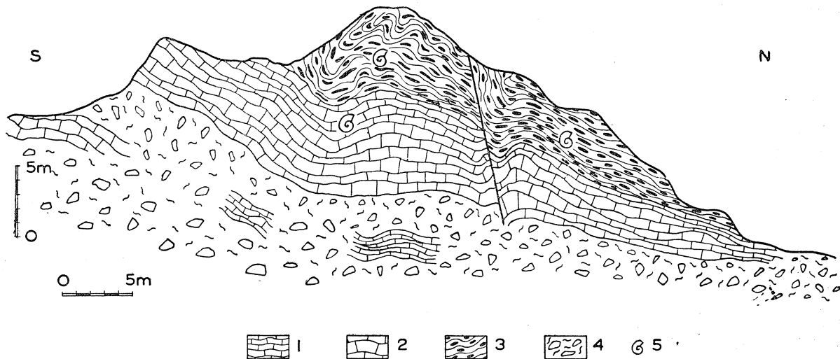
Fig. 2. Szkic geologiczny zachodniej ściany kamieniołomu. 1 — ciemnoczerwone wapienie cienko uławiczone; 2 — wapienie ciemnoczerwone grubo uwarstwione; 3 — łupki ilaste węglanowe z kongrecjami i bułami wapieni zawierającymi kolonie tabulatów i Cambrotrypa sudetica ; 4 — zwietrzelina; 5 — warstwy z fauną Fig. 2. Geological sketch of the western face of the quarry. 1 — dark-grey thin-bedded limestones; 2 — dark-grey thick-bedded limestones; 3 — clayey-carbonate shales with limestone concretions containing colonies of Cambrotrypa sudetica ; 4 — weathered rubble; 5 — fossiliferous beds
