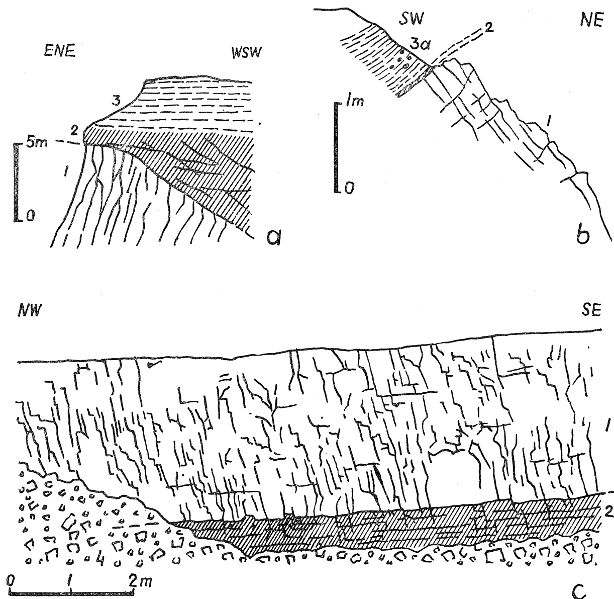
Fig. 8. a. Intruzyjny kontakt stropowy spilitu z łupkami dolnopermskimi w Świerkach-I (nowy kamieniołom) — depresja śródsudecka b. Intruzyjny kontakt stropowy spilitu z osadami dolnopermskimi w Świerkach-I (stary kamieniołom) — depresja śródsudecka c. Intruzyjny kontakt spągowy dolerytu kwarcowego z osadami dolnopermskimi w Świerkach-I (stary kamieniołom) — depresja śródsudecka Objaśnienia oznaczeń: 1 — doleryt-spilit; 2 — przeobrażone łupki; 3 — niezmienione łupki (3a — z kongrecjami marglistymi); 4 — usypisko
