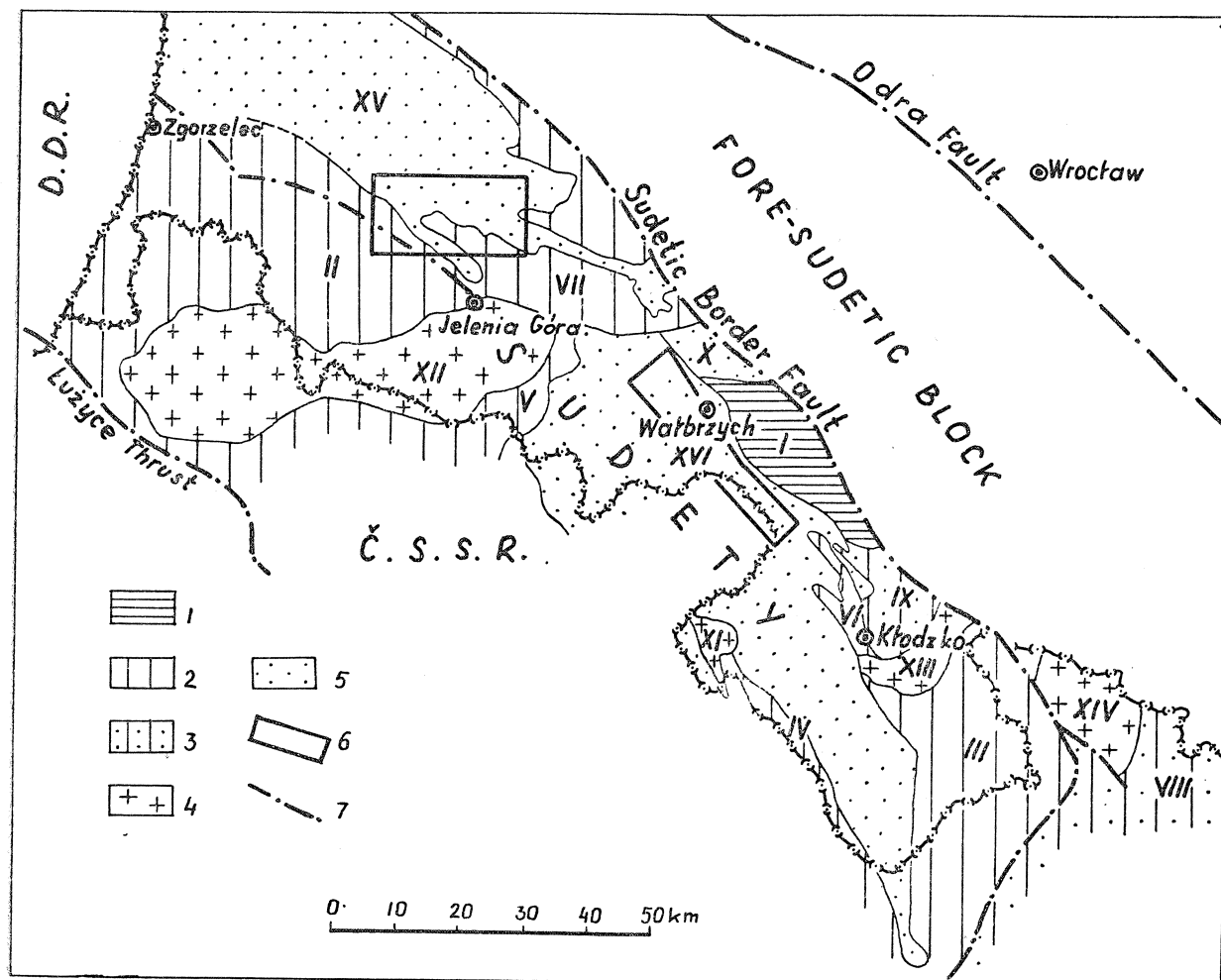
Fig. 1. Główne elementy strukturalne Sudetów (budowę geologiczną bloku przed-sudeckiego pominięto). 1 — skały archaiczne; 2 — skały prekambryjskie i staropaleozoiczne; 3 — skały paleozoiczne; 4 — granitoidy waryscyjskie; 5 — skały młodopaleozoiczne i mezozoiczne; 6 — obszary pobrania prób; 7 — główne dyslokacje; I — blok gnejsowy Gór Sowich; II — blok Karkonoszy—Gór Izerskich; III — kompleks metamorficzny Łądko-Snieżnika; IV — kompleks metamorficzny Gór Bystrzyckich i Gór Orlickich; V — kompleks metamorficzny wschodnich Karkonoszy; VI — kompleks metamorficzny kłodzki; VII — kaledonidy Gór Kaczawskich; VIII — struktura wschodniosudecka; IX — struktura Barda; X — depresja Świebodzić; XI — granitoidy Kudowej; XII — granitoidy Karkonoszy; XIII — intruzja kłodzko-ziotostocka; XIV — granitoidy Žulovej; XV — depresja północnosudecka; XVI — depresja śródsudecka
