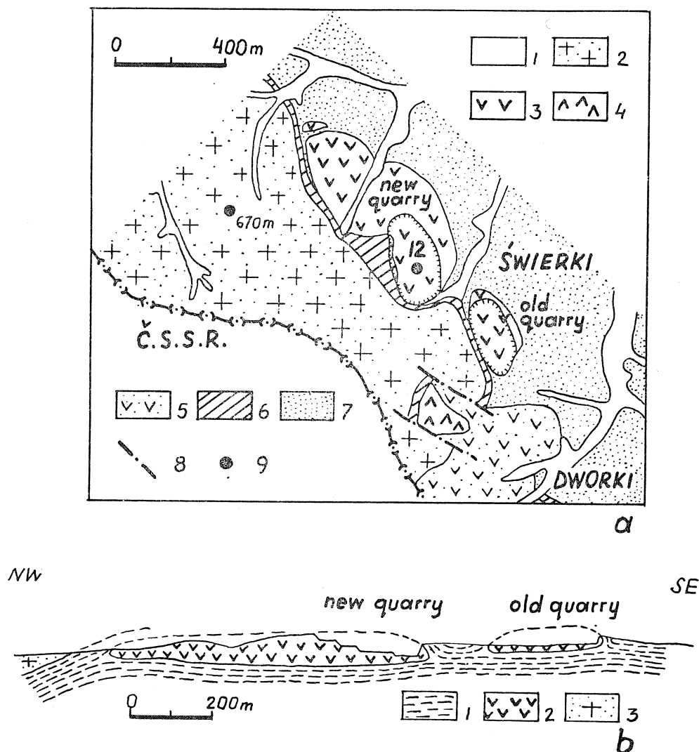
Fig. 7. a. Odsłonięcia skał dolnopermskich w Świerkach — depresja śródsudecka (budowa geologiczna uproszczona według Kozłowskiego, 1958, tabl. III). 1 — osady napływowe; 2 — porowaty porfir kwarcowy; 3 — doleryt-spilit itd. (skały intruzyjno-metasomatyczne, „melafirowe”); 4 — melafir wylewny; 5 — tuf melafirowy; 6 — łupki; 7 — piaskowiec „budowlany”: piaskowce i łupki (2—7 — czerwony spagowiec); 8 — uskoki; 9 — miejsca pobrania próbek
