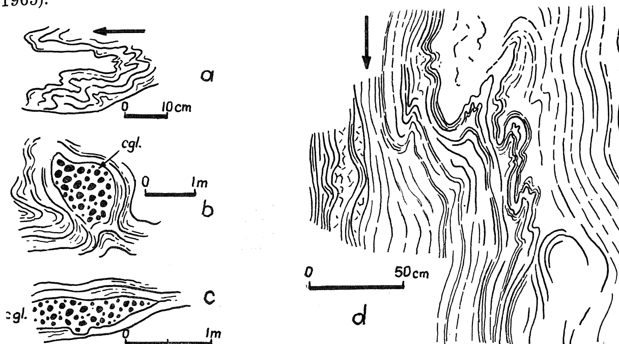
Fig. 11. a—c. Struktury fluidalne w wylewnym porfirze (westfal B/C) na górze Barbarka w depresji śródsudeckiej. d. Struktury fluidalne w wylewnym porfirze (górny westfal) w Starym Lesieńcu, w depresji śródsudeckiej. Cgl — zlepienie; strzałki wskazują kierunek płynięcia lawy porfirowej
