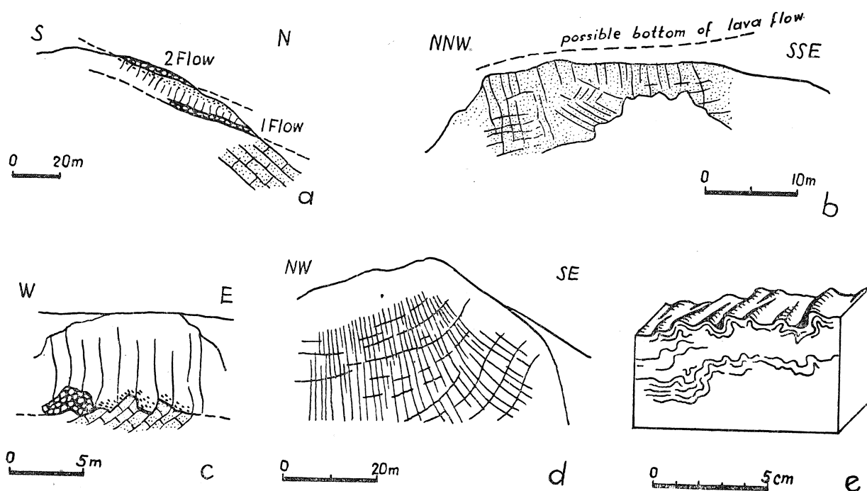
Fig. 5. Schematyczne profile geologiczne odsłoneń dolnopermskich law melafirowych, zmienionych osadów i wylewnego porfiru w depresji północnosudeckiej (skala przybliżona): a — Bełczyna; b — Sokołowiec; c — góra Rawka (Rząśnik); d — Wielisław Złotoryjski (porfir); e — Wielisław Złotoryjski, struktury fluidalne w porfirze. (Objaśnienia oznaczeń do fig. 5 a—c — jak na fig. 4)
