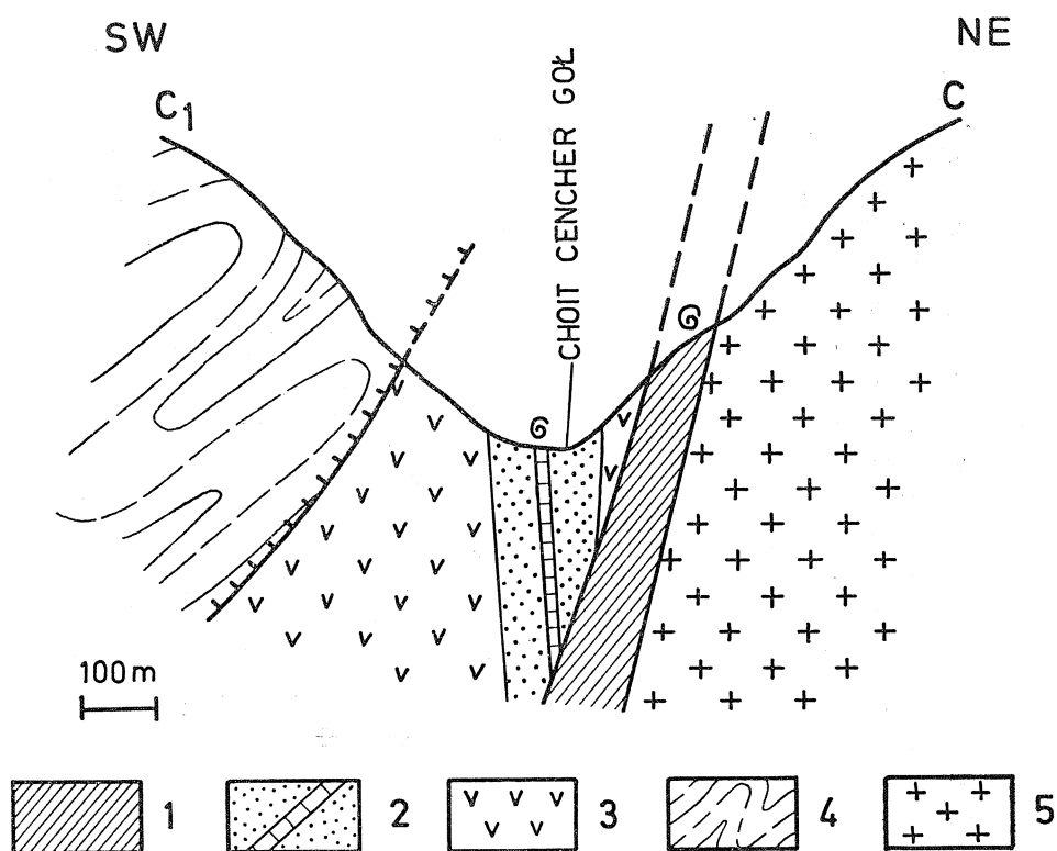
Fig. 5. Przekrój geologiczny przez dolinę Choit Cencher Goł 3,5 km poniżej ujścia Ulaan Goł. 1 — Sylur, łupki graptolitowe; Górny ordowik: 2 — piaskowce z wkładkami wapieni; 3 — porfiry; 4 — Seria górnoaltajska (ryfej górny — kambry dolny?); 5 — Granity późnokaledońskie
