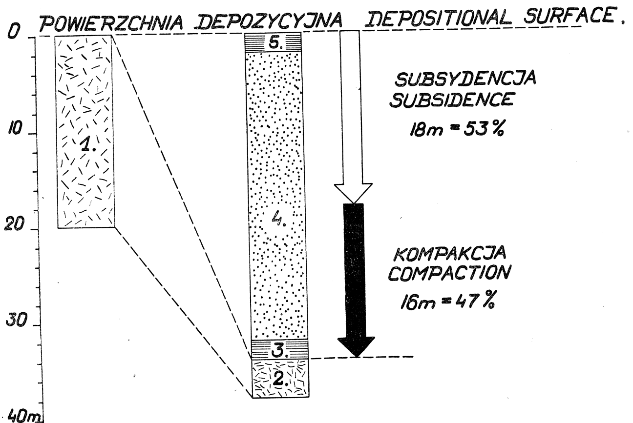
Fig. 21. Udział kompaktacji torfu i subsydencji w obniżaniu powierzchni depozycyjnej w fazie akumulacji osadów klastycznych na przykładzie cyklotemu modalnego ECAC. Nie uwzględniono kompaktacji osadów klastycznych. 1 — torf, zawartość wody 90%, miąższość 20 m; 2 — węgiel brunatny, zawartość wody 50%, miąższość 4 m; 3 — iłowiec, miąższość 2 m; 4 — piaskowiec gruboziarnisty miąższość 30 m; 5 — iłowiec, miąższość 2 m
