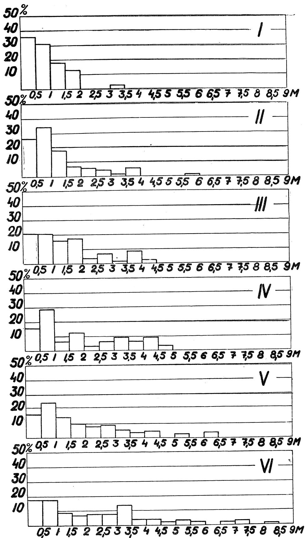
Fig. 10. Rozkłady miąższości pokładów węgla E. Na osi odciętych miąższość w m, na osi rzędnych częstość względna występowania. Węgiel pod piaskowcem gruboziarnistym A: I — cykle jednorodne; II — cykle proste; III — cykle złożone; węgiel pod iłowcem C: IV — cykle jednorodne; V — cykle proste; VI — cykle złożone
