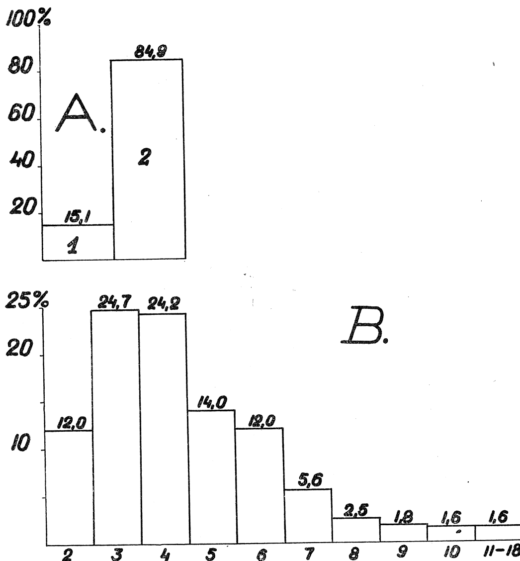
Fig. 5. Częstość cykli. A : 1 — cykle z ilowcem; 2 — cykle z piaskowcem. B — cykle z piaskowcem. Częstość w zależności od ilości elementów w cyklu przedstawionej na osi odciętych
