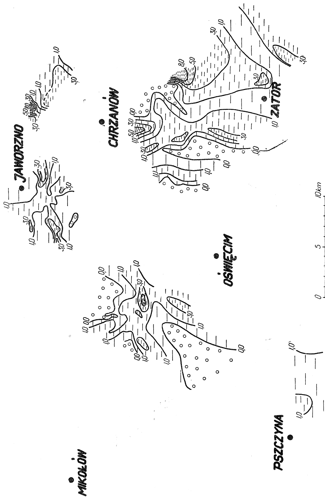
Fig. 13. Mapa miąższości ilowca w stropie pokładu 208. Oznaczenia jak na fig. 11
