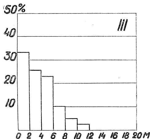
Fig. 8. Rozkłady miąższości ławic piaskowca drobnoziarnistego B. Na osi odciętych miąższość w m, na osi rzędnych częstość względna występowania. I — cykle jednorodne; II — cykle proste; III — cykle złożone
