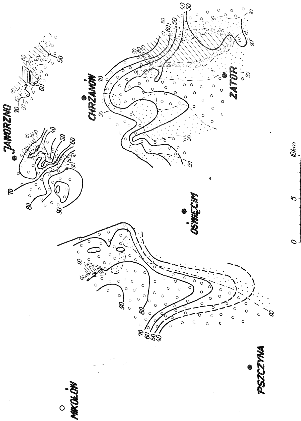
Fig. 17. Mapa miąższości i zapiaśszczenia cyklotemu między pokładami węgla 208—207. Oznaczenia jak na fig. 14 Fig. 17. Map of thickness and sandstone percentage in the cyclothem between the coal seams 208—207. For explanations see Fig. 14
