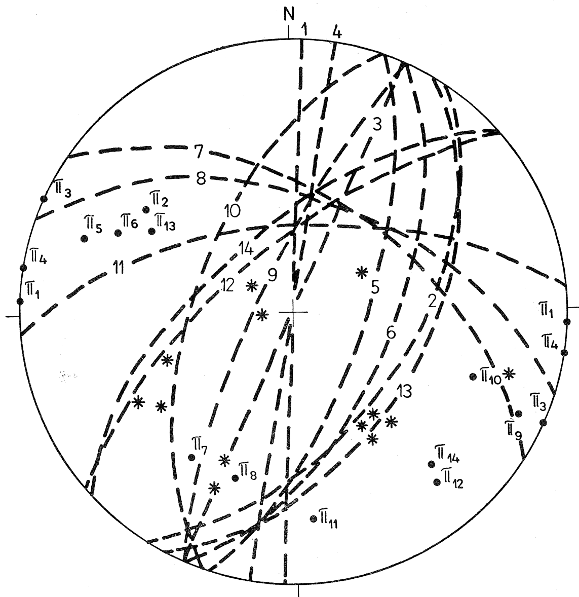
Fig. 13. Diagram drobnych uskoków przecinających wapienie dolnego kambru w łomie „Miłek” (Wojcieszów, Góry Kaczawskie). Dolna półkula projekcji równopowierzchniowej. Kropki — bieguny \pi dla powierzchni uskokowych (1—14); linie przerywane — duże koła powierzchni uskokowych (1—14); gwiazdki — rysy na ślizgach uskokowych
