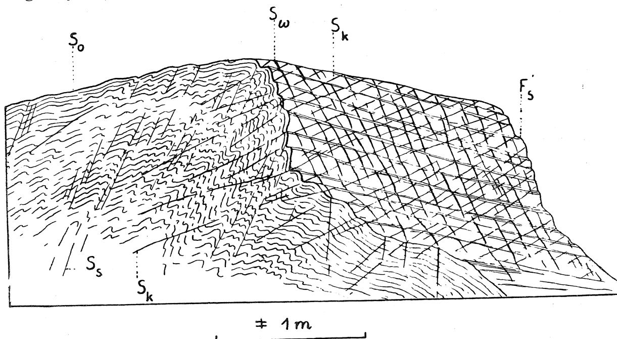
Fig. 1. Szklary — okolica na N od Międzygórza, grupa góriska Śnieżnika, drobnoziarniste gnejsy typu gieraltowskiego. F_s — fałd drobny systemu Śnieżnika (struktura główna); F_{s1}' — drobne fałdki na strukturze głównej; S_o — foliacja; S_{s1}' — złupkowanie spękania, związane z F_{s1}' ; S_k — złupkowanie spękania systemu Krowiarek; S_w — złupkowanie spękania systemu Wilczki
