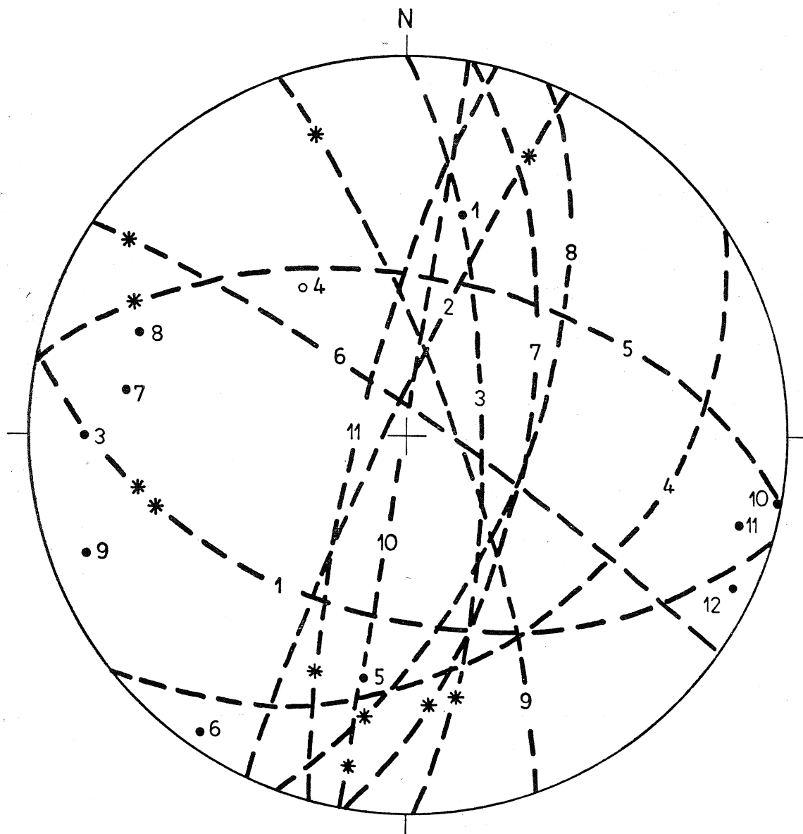
Fig. 15. Diagram drobnych uskoku, obserwowanych w łupkach zielenicowych jednostki Dobromierza wzdłuż doliny Strzegomki na S od Pietrzykowa. Projektacja równopowierzchniowa dolna półkula. Kropki — biegunki \pi dla powierzchni ślizgowych uskoku (1—12); duże koła (linie przerywane) — powierzchnie ślizgowe uskoku (1—12); gwiazdki — rysy na powierzchniach ślizgowych uskoku
