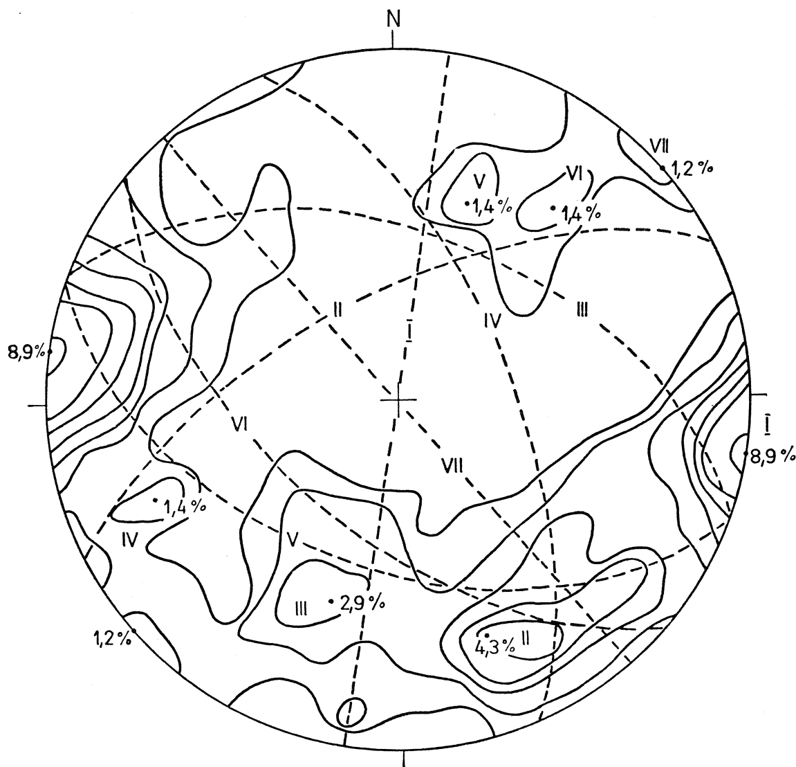
Fig. 14. Kumulatywny diagram dla 416 spękań skalnych pomierzonych w łupkach zieleńcowych jednostki Dobromierza w Pietrzykowie nad potokiem Strzegomka, bezpośrednio na S od wsi. Kontury 0,5, 1, 2, 3, 4, 5, 8% dla biegunów \pi powierzchni spękań. I—VII maksima zagęszczenia biegunów powierzchni spękań i odpowiadające im duże koło. Maksimum I odpowiada spękaniami równoległym do walnej dyslokacji N-S, biegnącej tu wzdłuż osi doliny Strzegomki. Maksima II, III, IV, V, VI i VII równoległe do drobnych uskoków zaznaczonych w intersekcji mapy i dostrzegalnych w odkrywkach
