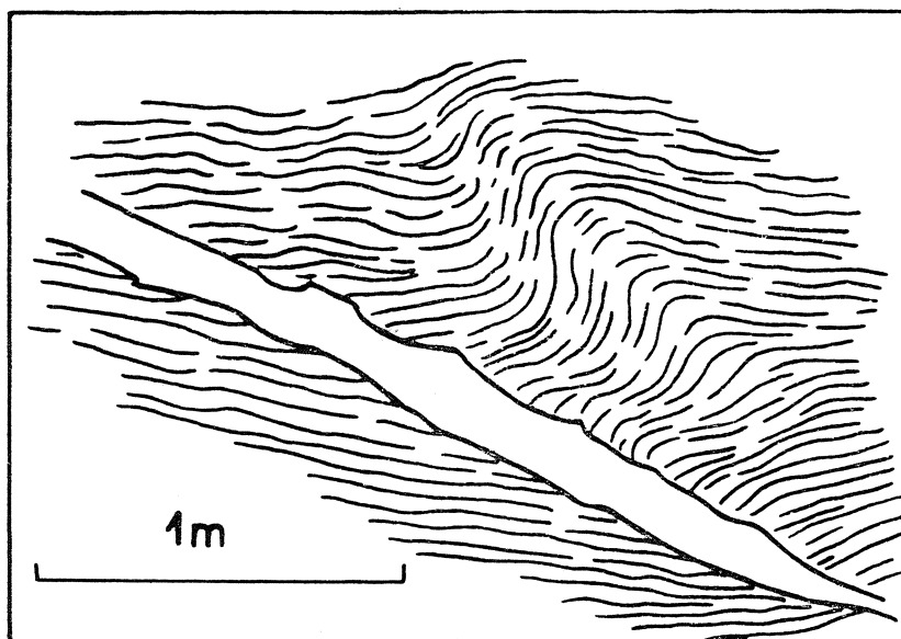
Fig. 8. Fałd w gnejsach drobnoziarnistych typu gieraltowskiego z żyłą kwarcu równoległą do powierzchni osiowej fałdu (łupki łyszczykowe w grupie górskiej Śnieżnika)
