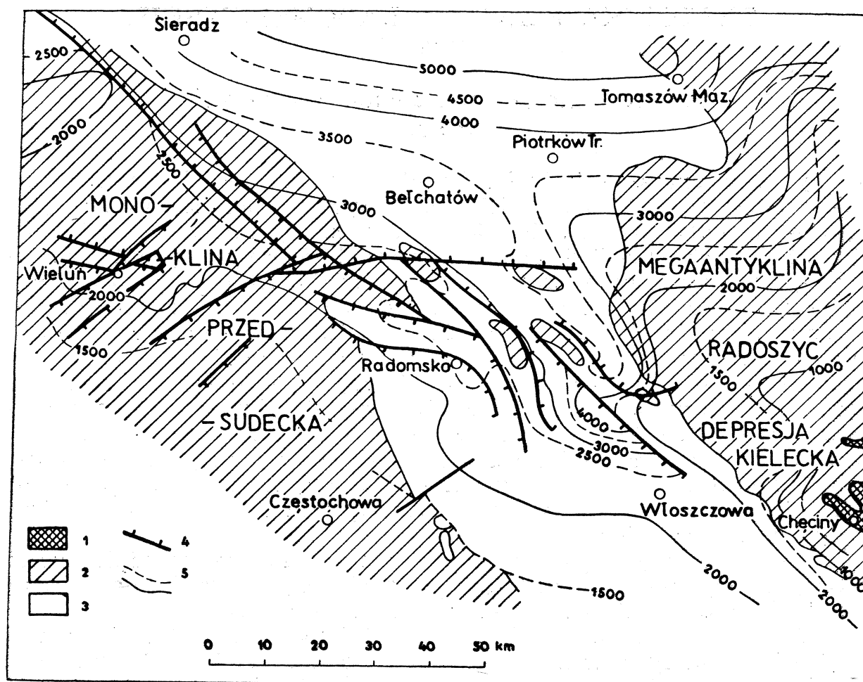
Fig. 1. Szkic głównych elementów tektonicznych elewacji radomskiej. 1 — wychodnie osadów paleozoiku; 2 — wychodnie jury pod kenozoikiem; 3 — wychodnie kredy pod kenozoikiem; 4 — dyslokacje; 5 — izolinie głębokości spagu cechsztynu Fig. 1. Sketch-map of principal tectonic elements of the Radomsko elevation. 1 — exposures of Paleozoic rocks; 2 — exposures of Jurassic rocks under the Cainozoic cover; 3 — exposures of Cretaceous rocks under the Cainozoic cover; 4 — faults; 5 — isolines of depth of the base of Zechstein
