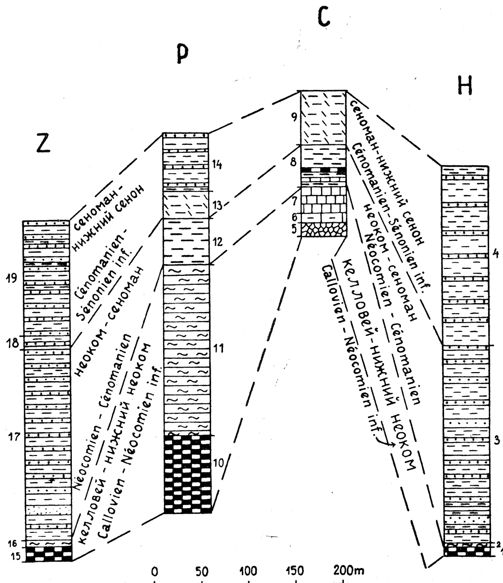
Фиг. 3. Разрезы утёсовых сукцессий в период келловей — нижней части верхнего мела. Колонки Р и С по данным К. Биркенмаера. Н — хулинская сукцессия: 1 — радиоларитовая серия; 2 — роговиковый известняк; 3 — „черный флиш”; 4 — пестрый флиш; С — чорштынская сукцессия в узком смысле: 5 — конкреционный чорштынский известняк (амонитико rosso); 6 — калпионелловые известняки и сопровождающие фации; 7 — брахиоподовые и криноидные известняки и сопровождающие фации; 8 — глобигериново-радиолариевые мергели и известняки; 9 — глоботрункановые пестрые мергели; Р — пенинская сукцессия в узком смысле: 10 — радиоларитовая серия; 11 — роговиковый известняк; 12 — глобигериново-радиолариевые мергели; 13 — пестрые мергели; 14 — тонкослоистый серый флиш; Z — златнянская сукцессия: 15 — радиоларитовая серия; 16 — роговиковый известняк; 17 — черный флиш; 18 — пестрый флиш; 19 — серый флиш Fig. 3. Profils des successions des Klippes depuis le Callovien jusqu'à partie inférieure du Crétacé supérieur. Colonnes P et C d'après les données de K. Birkenmajer. H — Succession de Hulina: 1 — radiolarites; 2 — calcaire à silex; 3 — flysch noir; 4 — flysch bigarré; C — succession de Czorsztyn (sensu stricto): 5 — calcaire noduleux de Czorsztyn („ammonitico rosso”); 6 — calcaires à Calpionelles et faciès qui les accompagnent; 7 — calcaires à Brachiopodes calcaires à Crinoides et faciès les accompagnant; 8 — marnes et calcaires à Globigérines et à Radiolaires; 9 — marnes bigarrées à Globotruncanes; P — succession des Pieniny (sensu stricto): 10 — radiolarites; 11 — calcaire à silex; 12 — marnes à Globigérines et à Radiolaires; 13 — marnes bigarrées; 14 — flysch gris à bancs minces; Z — succession de Zlatne; 15 — radiolarites; 16 — calcaire à silex; 17 — flysch noir; 18 — flysch bigarré; 19 — flysch gris
