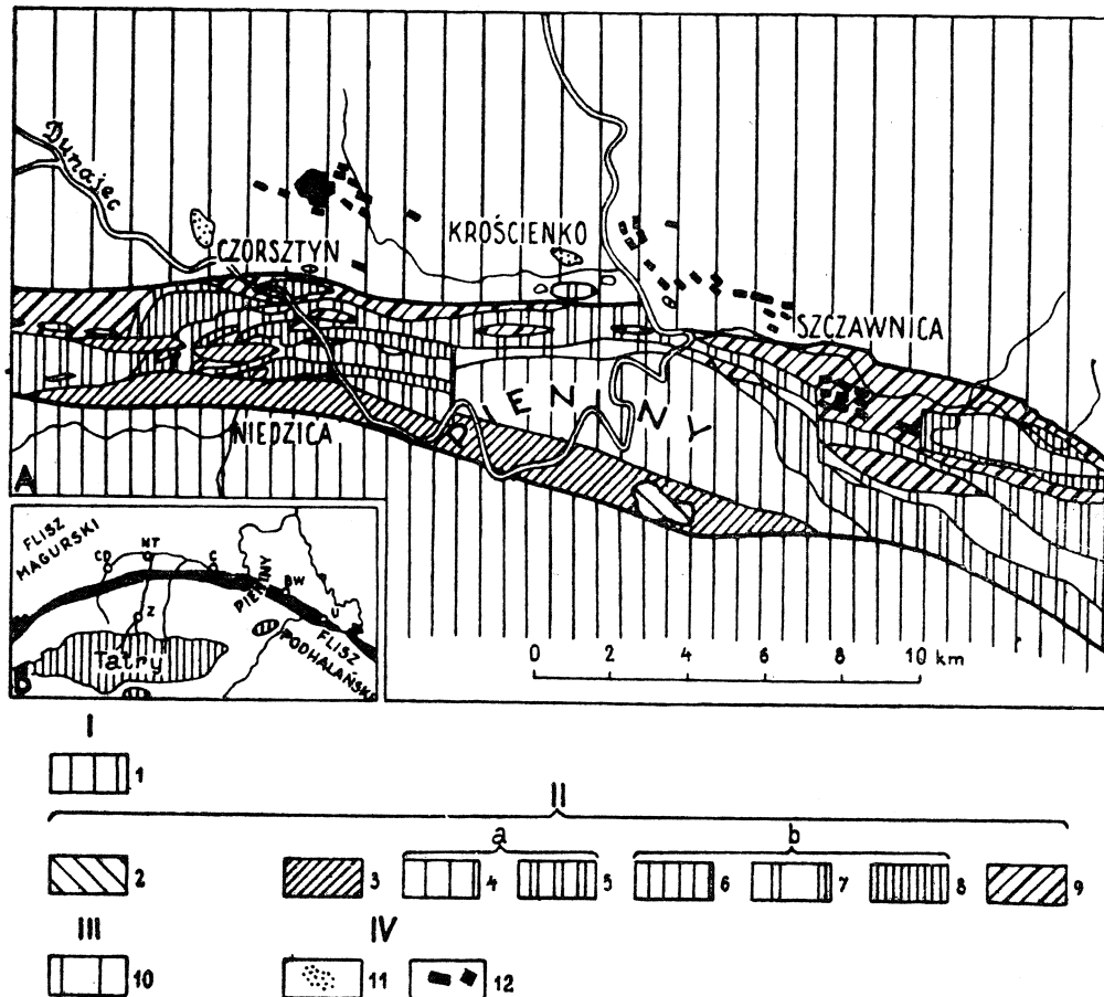
Фиг. 2а. Расположение утёсовых сукцессий в восточной части утёсовой зоны, находящейся на территории Польшы и на прилегающей части Словакии (частично по К. Биркенмаеру, 1959а). I — Внутренние Карпаты (интерниды): 1 — под-галлянский флиш; II — Пенинская утёсовая зона: 2 — галиговецкая сукцессия; 3 — златнянская сукцессия; 4 — пенинская сукцессия в узком смысле; 5 — браниская сукцессия (4 и 5 пенинская сукцессия в широком смысле); 6 — недзичкая сукцессия; 7 — чертезицкая сукцессия; 8 — чорштынская сукцессия (6, 7 и 8 чорштынская сукцессия в широком смысле); 9 — хулинская сукцессия; III — Внешние Карпаты (Флишевые): 10 — магурский покров; IV: — 11 — пресноводный неоген межгорных впадин; 12 — андезиты неогена
