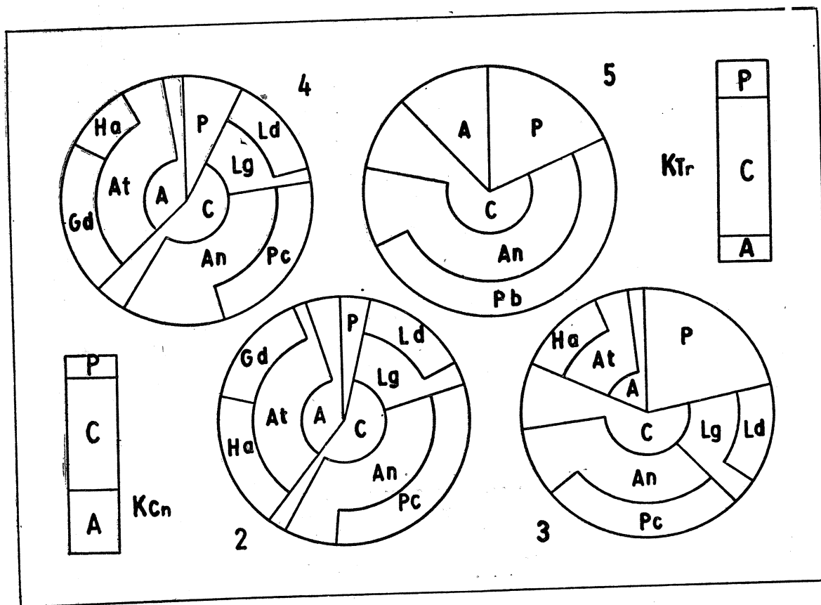
Fig. 2. Wykresy ilościowe składu zespołów otwornic z Raciborowic. KCn — zespół otwornic górnego cenomanu; KTr — zespół otwornic dolnego turonu; 2, 3, 4, 5 — zespoły otwornic z warstw 2—5. A — otwornice bentoniczne aglutynujące; B — otwornice bentoniczne wapienne; P — otwornice planktoniczne; Lg — Lagenidae ; Ld — Lenticulina ; An — Anomalinidae ; Pc — Pseudovalvulineria cenomanica ; Pb — Pseudovalvulineria berthelini ; At — Ataxophragmidae ; Ha — Hagenovella advena ; Gd — Gaudryina
