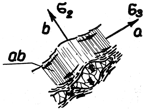
Fig. 2. Wzrost parakinematyczny soczewki porfiroblastu skalenia i jego wpływ na kierunek przemieszczeń biotyty w sąsiedztwie Fig. 2. Parakinematic growth of a feldspar porphyroblast lense and its influence on the direction of biotite displacement
