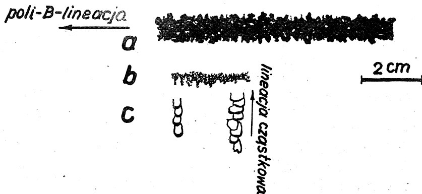
Fig. 1. a — prostolinijne skupienia złożonej lineacji biotyty (poli-B-lineacja); b — strzępiaste zakończenia poli-B-lineacji biotyty; c — lineacja cząstkowa z przedstawionym kierunkiem względnych przemieszczeń
