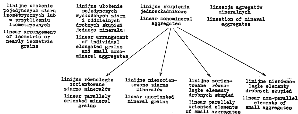
Fig. 1. Mezoskopowe typy B-lineacji ziarna Fig. 1. Types of mesoscopic B-lineation of mineral grains
