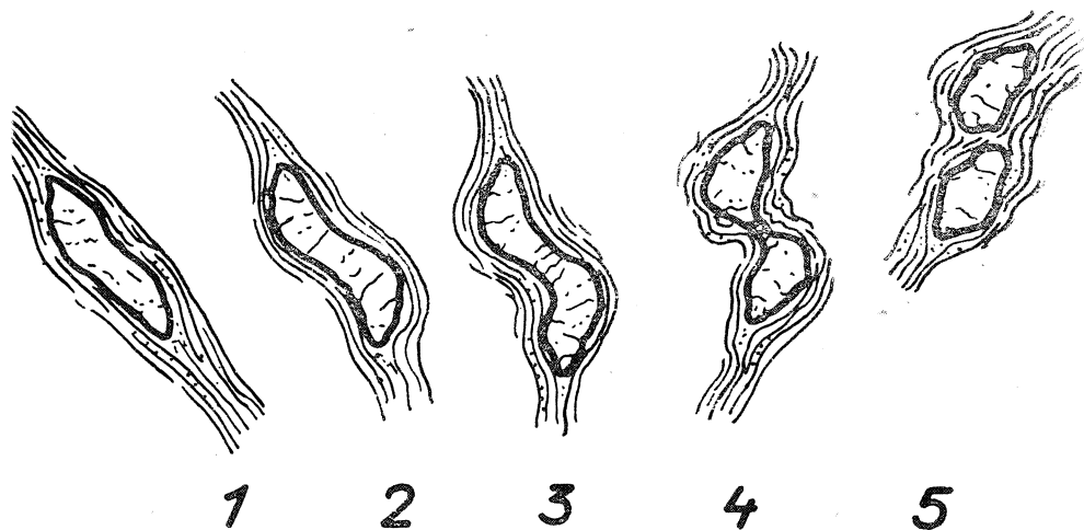
Fig. 8. Etapy rozrywania soczewek skaleniowych w gnejsach okolic Gryfowa Śląskiego Fig. 8. Phases of deformation of feldspar lenses in gneisses, Gryfów Śląski area
