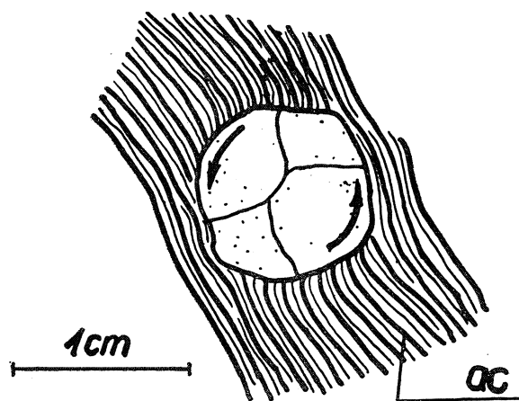
Fig. 4. Rotacja ziarna granatu w łupkach łyszczykowych (okolicy Krobicy) Fig. 4. Rotation of a garnet grain in mica-schists. Krobica area
