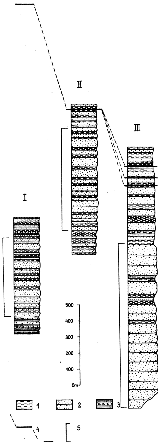
Fig. 1. Profile dolnych warstw krośnieńskich. 1 — łupki i cienkoławicowe piaskowce; 2 — grubo- i średnioławicowe piaskowce przykładane łupkami; 3 — warstwy menilitowe i przejściowe; 4 — położenie korelacyjnego poziomu łupków jasielskich; 5 — opróbowane odcinki profili; I — profil proksymalny regionu I (Gorlice, dolina Ropy); II — profil proksymalny regionu II (Zagórz, dolina Oslawy); III — profil proksymalny regionu III (Ustrzyki Górne, dolina potoku Wołosatego)
