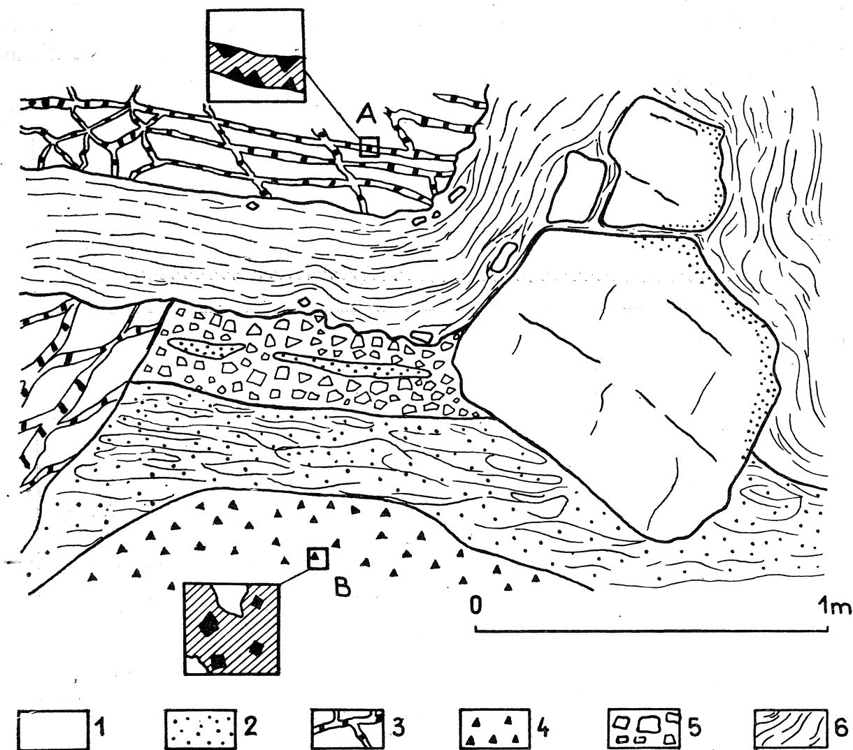
Fig. 4. Przykład wykształcenia utworów brekcyjowych: 1 — dolomit kruszonośny; 2 — rozsypliwy dolomit; 3 — żyły kalcytowe z galeną; 4 — gniazda kalcytowe impregnowane galeną; 5 — brekcja dolomitowa spojona kalcytem; 6 — zielone ily (liniami zaznaczono przebieg powierzchni nieciągłości); mineralizacja galenowa w żyłach (A) i gniazdach (B) kalcytowych: galena (czarna), kalcyt (zakreskowany), dolomit (biały)
