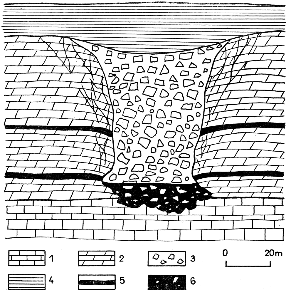
Fig. 6. Okruszcowanie w jamach krasowych: 1 — wapienie gogolińskie; 2 — dolomity kruszczońskie i diploporowe; 3 — brekcje; 4 — iły tortońskie; 5 — horyzonty rudne w dolomitach kruszczońskich; 6 — okruszcowane brekcje
