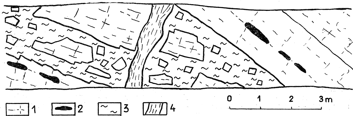
Fig. 3. Przykład wykształcenia utworów brekcjowych: 1 — bloki dolomitu; 2 — konkracje krzemionkowe; 3 — brązowe iły piaszczyste i drobnoziarniste brekcje; 4 — zielone iły (liniami zaznaczono przebieg powierzchni nieciągłości)
