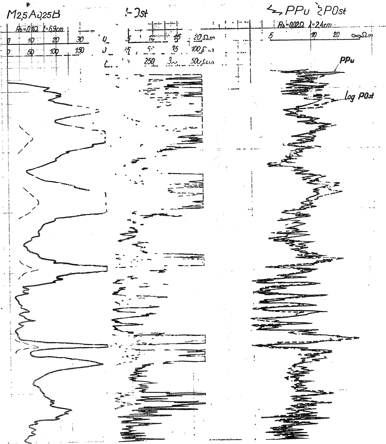
Фиг. 4. Сопоставление кривой каротажа проводимости КП с комплектом геофизических данных; Post — БК; PPu — КПб
