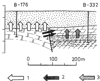
Fig. 9. Przekrój geologiczny ilustrujący niektóre typy kontaktów hydraulicznych na południe od Bolesławia. 1 — strefa kontaktu erozyjnego (IB2) piętra wodonośnego czwartorzędowego z dewońskim; 2 — strefa kontaktu tektonicznego (IB1) piętra wodonośnego triasowego z dewońskim; 3 — strefa kontaktu metasomatycznego (IB4) poziomego wodonośnego wapienia muszlowego i retu. Objasnienia geologiczne jak na fig. 7
