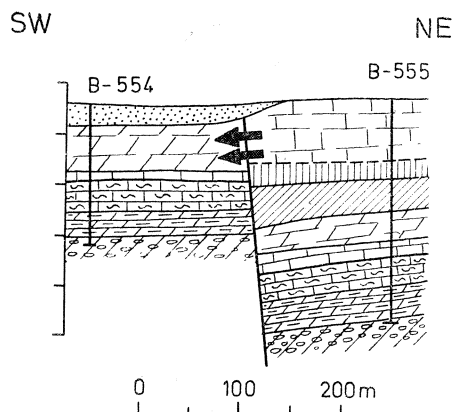
Fig. 10. Przykład kontaktu hydraulicznego typu tektonicznego (IB1) pomiędzy jurajskim i triasowym piętrem wodonośnym w rejonie Klucz. Strzałkami pokazano strefę kontaktu. Objasnienia geologiczne jak na fig. 7
