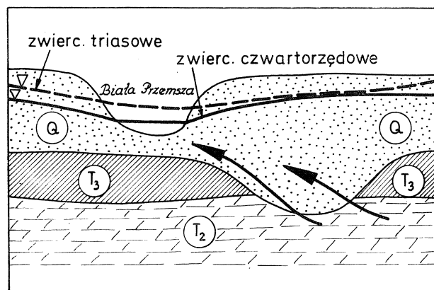
Fig. 15. Szkic ilustrujący strefę rozładowania ciśnienia naporowego horyzontu triasowego w warunkach reżimu naturalnego. T 2 — wapień muszlowy, dolomity kruchości i diplopore; T 3 — kajper, seria ilasta; Q — czwartorzęd, piaski
