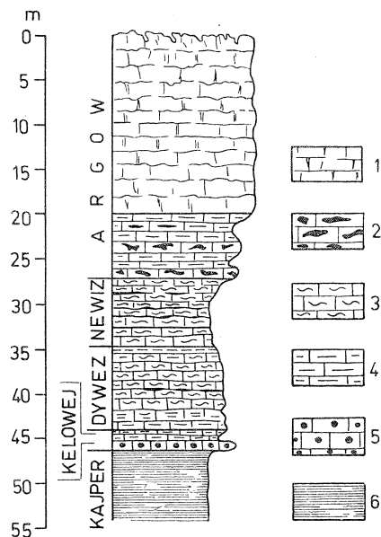
Fig. 4. Profil dolnej części jury przy drodze z Klucze do Olkusza (według S. Z. Różyckiego, 1953). 1 — wapienie płytowe; 2 — wapienie gąbkowe; 3 — margle ilaste; 4 — margle; 5 — wapienie oolitowe; 6 — iłolupki
