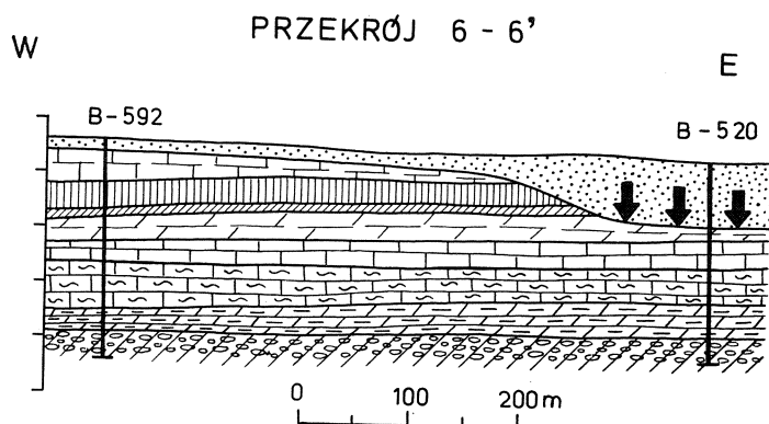
Fig. 12. Przykład kontaktu hydraulicznego typu erozyjnego (IB2) pomiędzy czwartorzędowo-jurajskim i triasowym piętrzem wodonośnym we wschodniej części rejonu olkuskiego. Strzałkami pokazano strefę kontaktu. Objaśnienia jak do fig. 7
