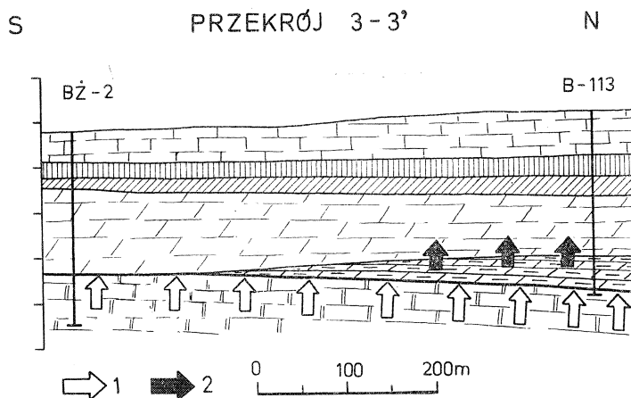
Fig. 5. Przekrój geologiczny ilustrujący niektóre typy kontaktów na południe od Olkusza. 1 — strefa kontaktu sedymentacyjno-transgresywnego (IA2) i metasomatycznego (IB4) piętra wodonośnego triasowego z dewońskim; 2 — strefa kontaktu metasomatycznego (IB4) pomiędzy wodonośnym poziomem wapienia muszlowego i retu. Objaśnienia geologiczne jak na fig. 7
