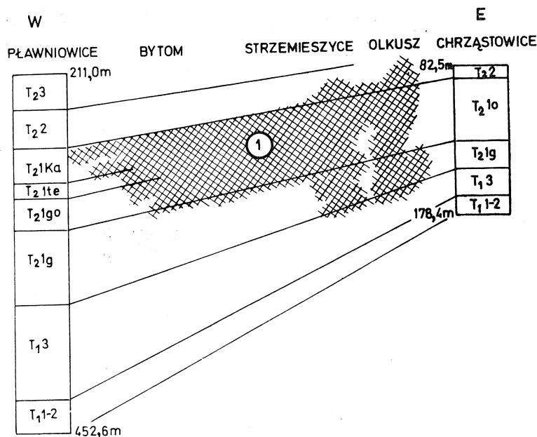
Fig. 13. Schematyczny przekrój geologiczny ilustrujący niezgodny stosunek dolomitów kruszconośnych do stratygrafii (według S. Sliwińskiego, 1969). T_{1-2} — niższy pstry piaskowiec; T_1^s — ret; T_2^1g — warstwy gogolińskie; T_2^1go — warstwy górażdzkie; T_2^{1te} — warstwy terebratulowe; T_2^{1ka} — warstwy karchowickie; T_2^2 — dolomity diploporowe; T_3 — kajper
