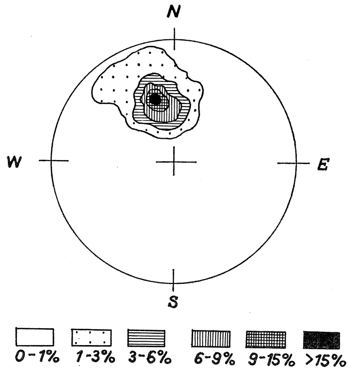
Fig. 4. Stereogram spękań S_0 . Fragment odkrywki w dolinie Mangusz. Pomiarów 257, półkula górna
