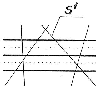
Fig. 5. Spękania S^1 (ścinające)
