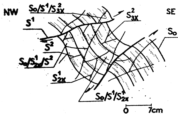
Fig. 26. Fragment odkrywki aleurytów i argilitów taurydzkiej serii położonej w dolinie Mangusz. Przekrój prostopadły do liniowych elementów skalnych ( B_s=27/46 ). Na rysunku liniowe elementy skalne są ograniczone spękaniem
