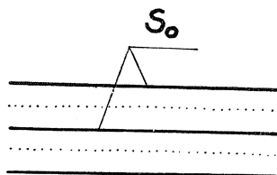
Fig. 3. Spękania S_0 ( ab ) równoległe do warstwowania
