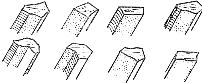
Fig. 1. Schematyczny rysunek różnych kształtów liniowych elementów skalnych w przekroju ac w argilitach i aleurytach taurydzkiej serii
