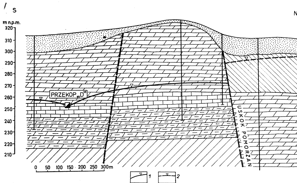
Fig. 14. Przekrój hydrogeologiczny przez uskoku Pomorzany w rejonie przekopu „D”: 1 — swobodne zwierciadło wody; 2 — naporowe zwierciadło wody (powierzchnia piezometryczna). Pozostałe objaśnienia jak na fig. 10
