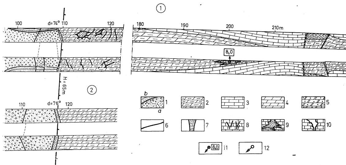
Fig. 4. Profile geologiczne 1 i 2 wzdłuż wyrobisk udostępniających złożę rudy: 1 — utwory permskie; a — zlepieńce, b — piaskowce (niższy pstry piaskowiec?); 2 — dolomityczno-margliste utwory retu; 3 — wapienie warstw gogolińskich i olkuskich; 4 — dolomity kruszczońskie; 5 — dolomity diploporowe; 6 — fuga międzyławicowa na kontakcie ret-wapienie gogolińskie; 7 — szczelina uskoku głównego wypełniona materiałem ilastym (niższy pstry piaskowiec?); 8 — szczeliny i spękania; 9 — kieszeń krasowa wypełniona materiałem; 10 — nie wypełnione kawerny krasowe; 11 — miejsca wystąpienia dużych wypływów z podaną wydajnością w m 3 /min; 12 — mniejsze wypływy i wycieki; 13 — przebieg uskóków
