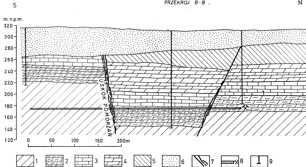
Fig. 10. Przekrój geologiczny przez uskók Pomorzany wzdłuż profilu 3: 1 — zlepienie permu; 2 — dolomityczno-margliste utwory retu z utworami niższego pstręgo piaskowca w spągu; 3 — wapienie dolnego wapienia muszlowego; 4 — dolomity kruszczone i dipoporowe (dolny i środkowy wapień muszlowy); 5 — ilaste osady kajpru; 6 — piaski czwartorzędowe; 7 — spękania strefy uskokowej; 8 — przekop polowy; 9 — otwory wiertnicze
