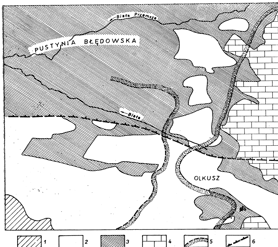
Fig. 1. Schematyczny szkic przebiegu uskoku Pomorzany na tle sytuacji hydrogeologicznej (wg. Z. Wilka i W. Zimnego, 1973): 1 — zasięg wychodni słabo przepuszczalnych zlepieńców permjskich; 2 — wychodnie triasowego piętra wodonośnego, wapień muszlowy i ret; 3 — nieprzepuszczalne utwory kajpru; 4 — wodonośne wapienie jury; 5 — schematyczne kontury pogrzebanej doliny wypełnionej piaskami rzecznotodowcowymi; 6 — schematyczny przebieg uskoku głównego Pomorzany
