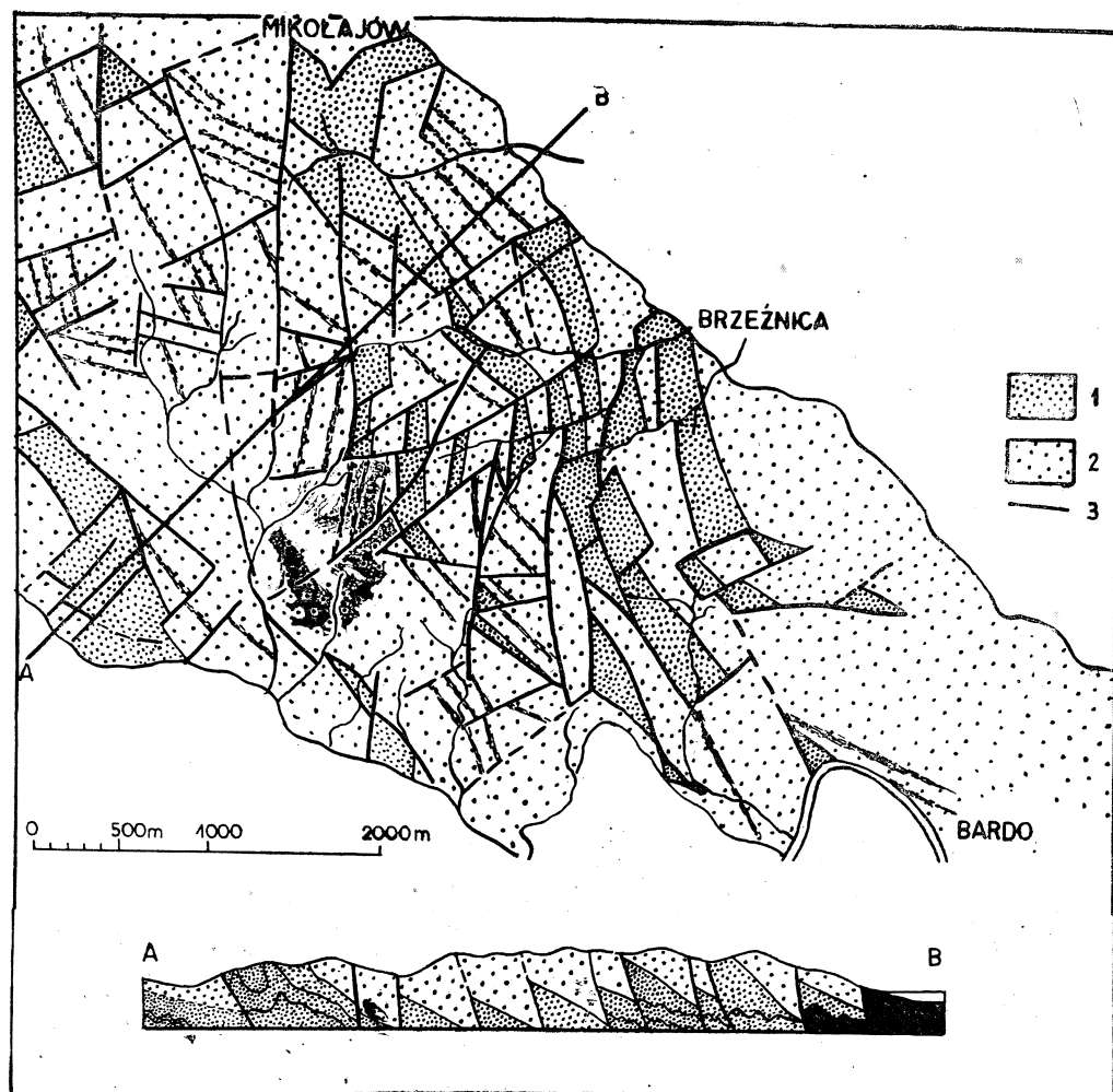
Fig. 5. Wycinek mapy geologicznej arkusza Zabkowice Śląskie i przekrój geologiczny (wg Finckha, 1926). 1 — utwory przedkarbońskie; 2 — utwory dolnego karbonu; 3 — uskoki
