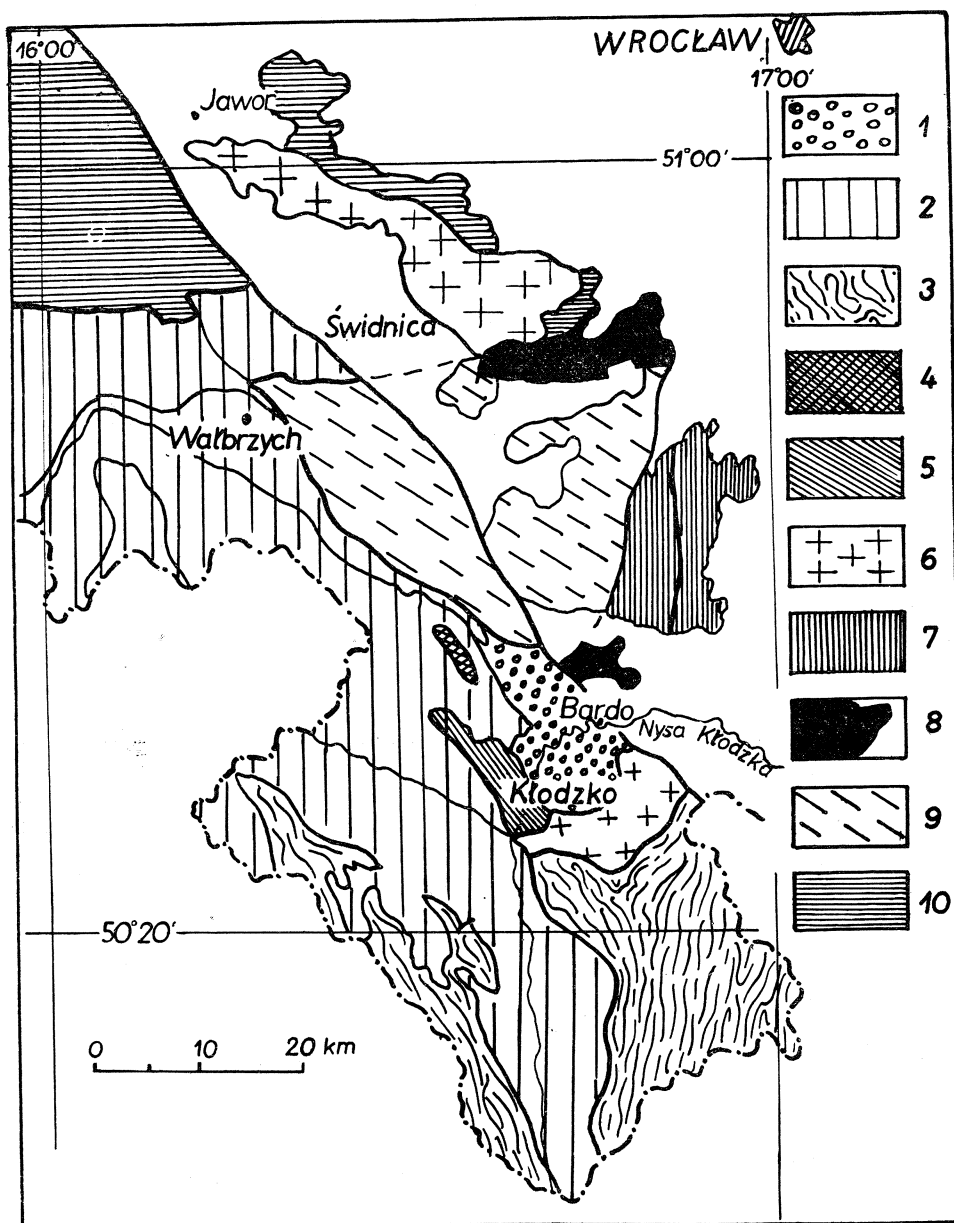
Fig. 1. Przeglądowa mapa geologiczna Sudetów środkowych (wg Sawickiego i Teisseyre'a, 1969; uproszczone). 1 — Góry Bardzkie; 2 — depresja śródsudecka (karbon, perm, trias i górna kreda); 3 — metamorfik Złotego Stoku; 4 — blok gabbro-diabazowy Nowej Rudy—Ślupca; 5 — metamorfik kłodzki; 6 — masywy granitoidowe; 7 — strefa Niemczy i metamorfik Kamieńca; 8 — serpentynity; 9 — gnejsowa kra Gór Sowich; 10 — epimetamorfik Gór Kaczawskich
