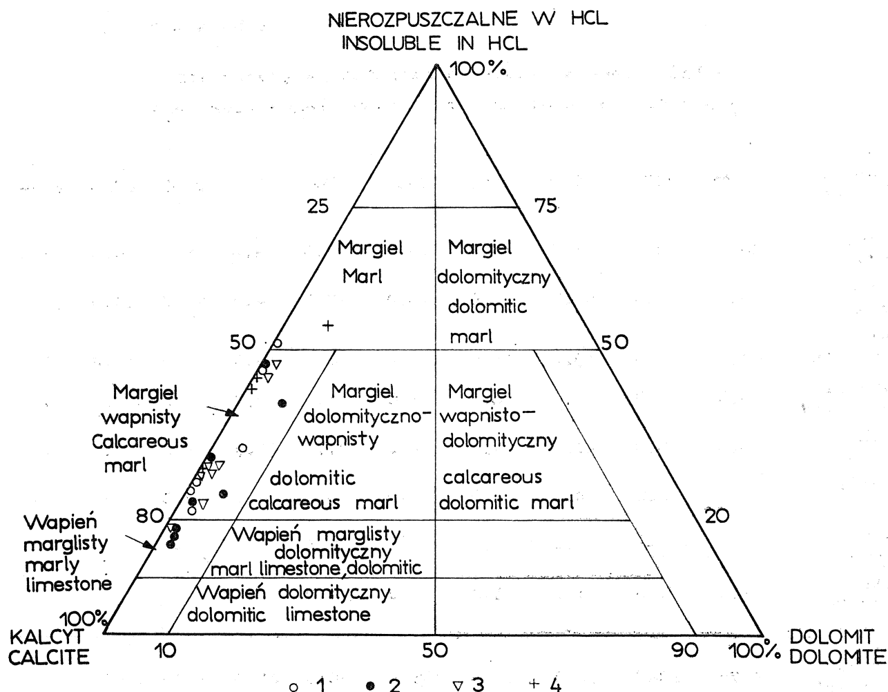
Fig. 2. Klasyfikacja margli
