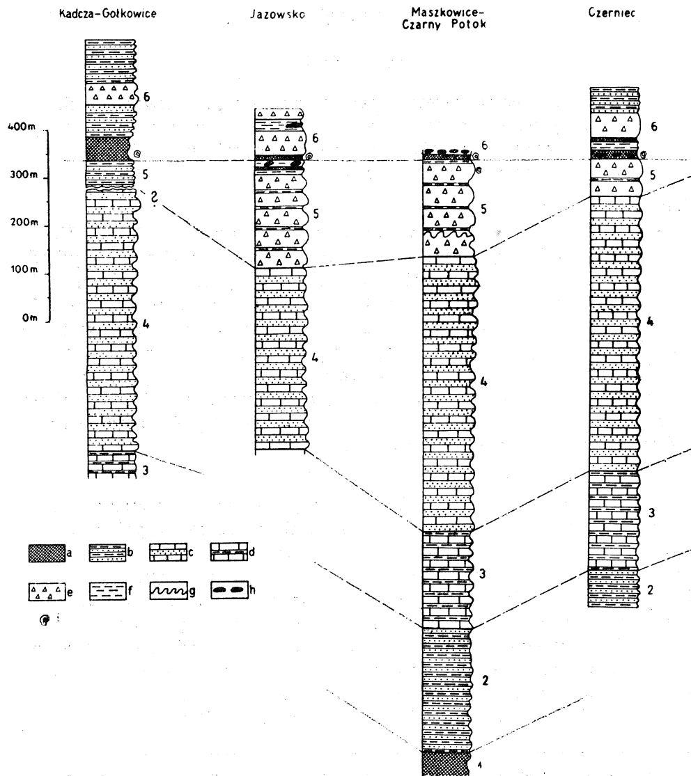
Fig. 3. Profile litostratygraficzne strefy sądeckiej. a — łupki pstre, b — piaskowce cienkoławicowe, łupki ilaste, c — piaskowce gruboławicowe, margle, d — piaskowce cienkoławicowe, łupki ilaste, margle, e — piaskowce gruboławicowe z fragmentami łupków, f — łupki zielone, g — osuwiska podmorskie, h — konkretacje manganowe, i — Cyclammina amplexans Grzybowski; 1 — łupki pstre, 2 — warstwy beloveskie, 3 — warstwy łackie dolne, 4 — warstwy łackie górne, 5 — warstwy z Maszkowic, 6 — warstwy z Jazowska
