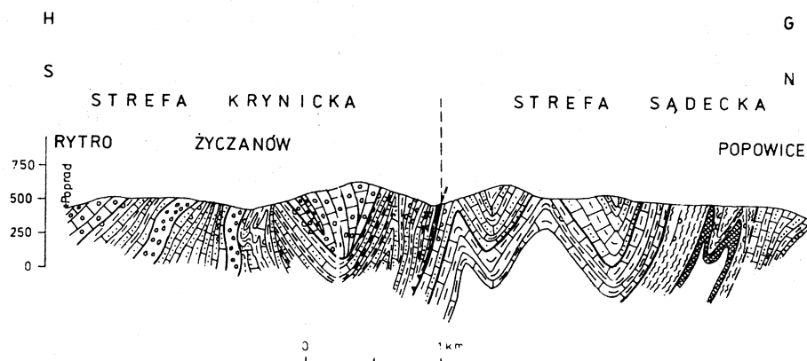
Fig. 10. Przekrój geologiczny G—H. Objaśnienia jak na fig. 7
