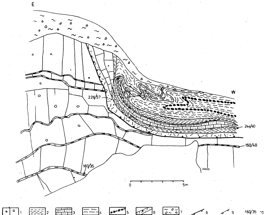
Fig. 4. Nasunięcie warstw z Jazowska na warstwy z Maszkowic w Łącko-Zawodzie. Warstwy z Maszkowic: 1 — piaskowce gruboławicowe z fragmentami łupków, 2 — łupki zielone, warstwy z Jazowska: 3 — piaskowce cienkoławicowe, 4 — łupki czerwone z Cyclamina amplexans Grzybowski, 5 — konkretne manganowe, 6 — brekcja tektoniczna — pokruszone piaskowce ze strzałką kalcytową, 7 — gliny zwietrzelinowe z rumoszem piaskowców, 8 — nasunięcie, 9 — położenie hieroglifów, 10 — kierunek zapadania warstw (kąt zapadania warstw)
