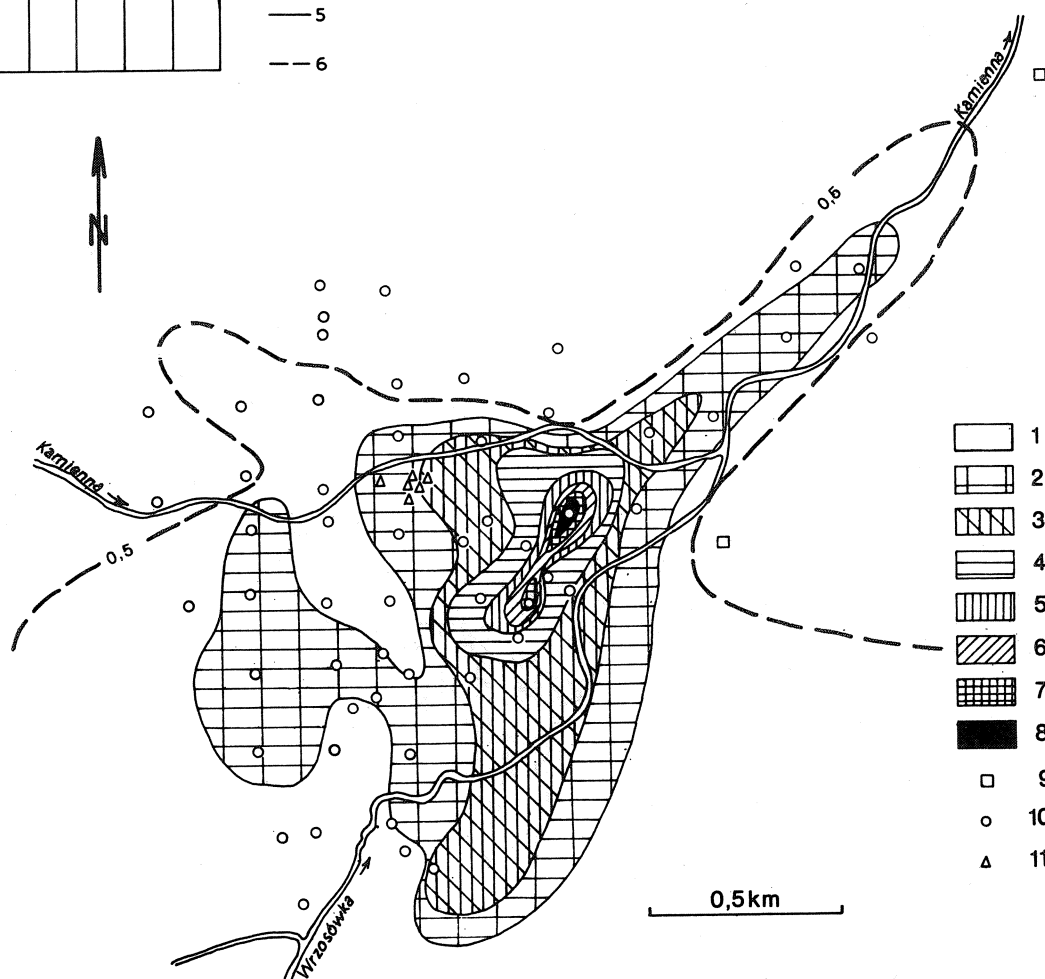
Fig. 3. Mapka koncentracji fluoru w wodach zwykłych Cieplic Śl. Zdroju. 1-8 - obszary występowania wód zawierających jon fluorowy w ilości (w mg/l): 1 - 0-1, 2 - 1-2, 3 - 2-3, 4 - 3-4, 5 - 4-5, 6 - 5-6, 7 - 6-7, 8 - >7; 9 - studnie; 10 - płytkie otwory wiertnicze; 11 - źródła termalne
