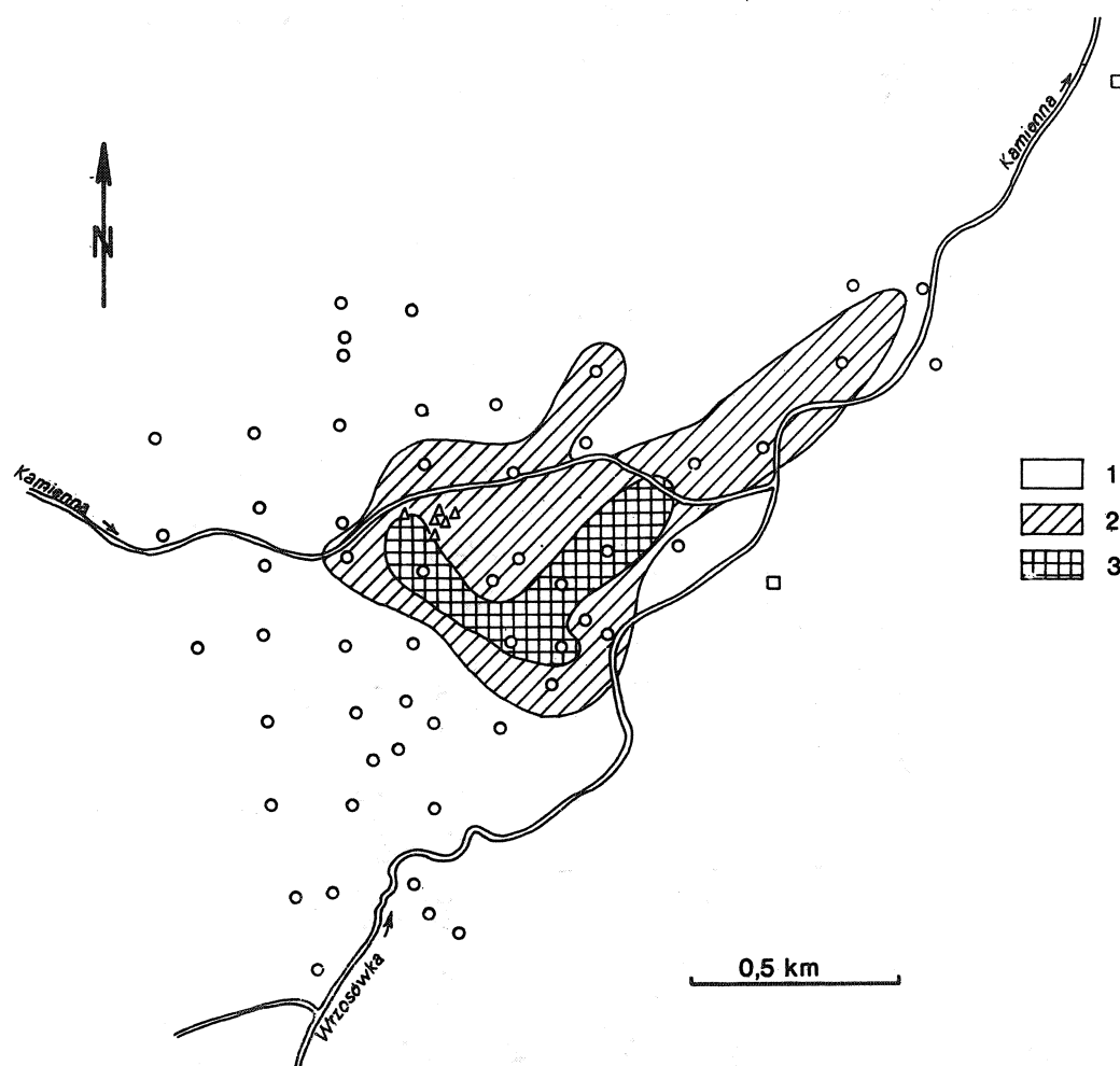
Fig. 5. Mapka koncentracji sodu w wodach zwykłych Ciepliec Śl. Zdroju. 1–3 – obszary występowania wód zawierających jon \text{Na}^+ w ilości (w mg/l): 1 – 0–50; 2 – 50–100; 3 – >100. Pozostałe objaśnienia jak na fig. 3
