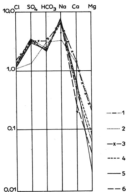
Fig. 2. Analizy chemiczne wód termalnych (z r. 1970) przedstawione na wykresie Schoellera. Zawartość jonów wyrażona w miliwalach. Ujęcia: 1 - Marysieńka, 2 - Sobieski, 3 - Wacław-Antoni, 4 - Nowe, 5 - basenowe (damskie), 6 - basenowe (męskie)
