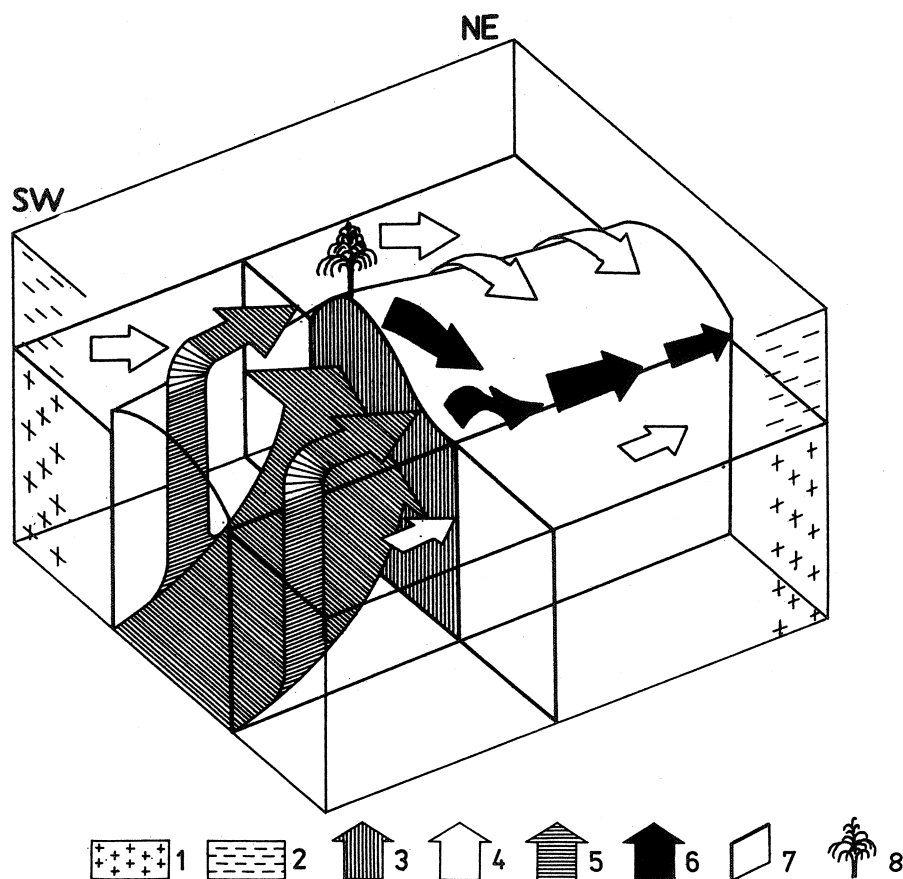
Fig. 9. Schemat tworzenia się anomalii hydrogeochemicznej Cieplic Śl.-Zdroju. 1 – granit, 2 – utwory czwartorzędowe, 3 – wody termalne typu \text{SO}_4-\text{HCO}_3-\text{Na} , 4 – wody zwykłe typu \text{SO}_4-(\text{HCO}_3-\text{Cl})-\text{Ca}-(\text{Mg}-\text{Na}) oraz \text{HCO}_3-(\text{SO}_4-\text{Cl})-\text{Ca}-\text{Na}-(\text{Mg}) , 5 – wody głębszego krążenia typu \text{HCO}_3-(\text{SO}_4)-\text{Na}-\text{Ca} , 6 – wody mieszane typu \text{HCO}_3-\text{SO}_4-(\text{Cl})-\text{Na}-(\text{Ca}) , 7 – strefy uskokuwe, 8 – źródła wód termalnych
