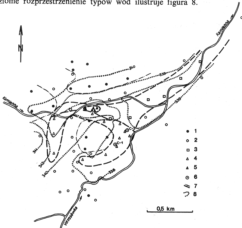
Fig. 8. Mapka hydrochemiczna obszaru Ciepliec Śl. Zdroju. 1-5 - typy wód: 1 - SO_4-(HCO_3-Cl)-Ca-(Mg-Na) , 2 - HCO_3-(SO_4-Cl)-Ca-Na-(Mg) , 3 - HCO_3-SO_4-(Cl)-Na-(Ca) , 4 - HCO_3-(SO_4)-Na-Ca , 5 - SO_4-HCO_3-Na (wody termalne oprócz źródła Sobieski), 6 - głębokie otwory wiertnicze, 7 - granice chemicznych typów wód, 8 - hydroizohipsy
