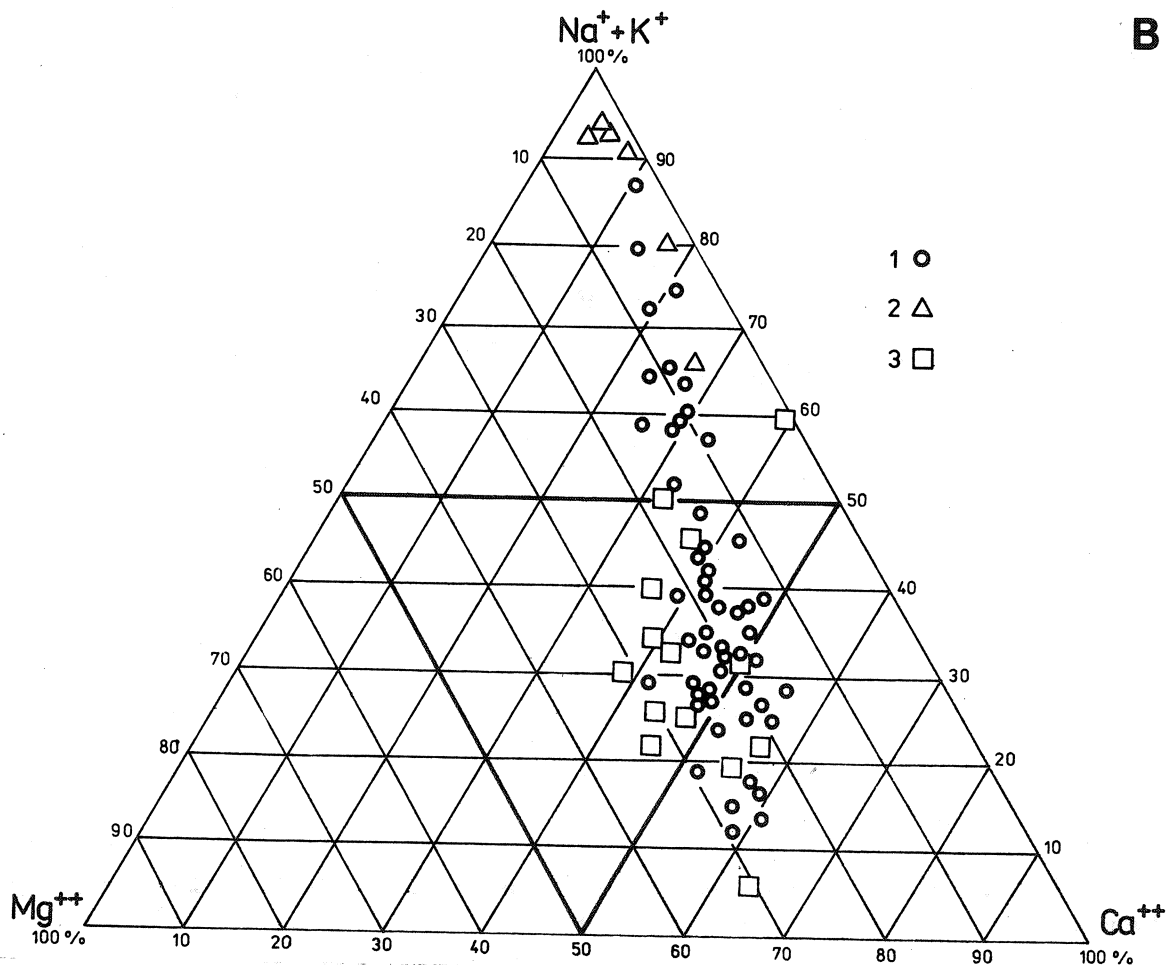
Fig. 6. Wykresy składu chemicznego wód termalnych i wód zwykłych z otworów płytkich, studni i źródeł. A – aniony, B – kationy. 1 – otwory płytke, 2 – źródła termalne, 3 – studnie i źródła Fig. 6. Diagrams of chemical composition of thermal and normal waters from shallow boreholes, wells and springs. A – anions, B – cations. 1 – shallow boreholes, 2 – thermal springs, 3 – wells and springs
