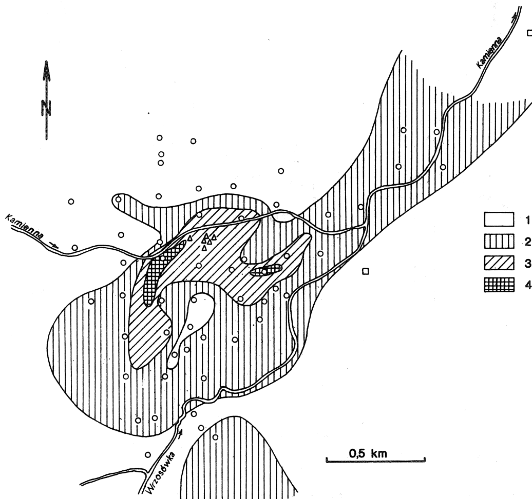
Fig. 4. Mapka koncentracji wodorowęglanów w wodach zwykłych Cieplíc Śl. Zdroju. 1-4 - obszary występowania wód zawierających jon HCO_3 w ilości (w mg/l ): 1 - 0-100; 2 - 100-200; 3 - 200-300; 4 - > 300. Pozostałe objaśnienia jak na figurze 3
