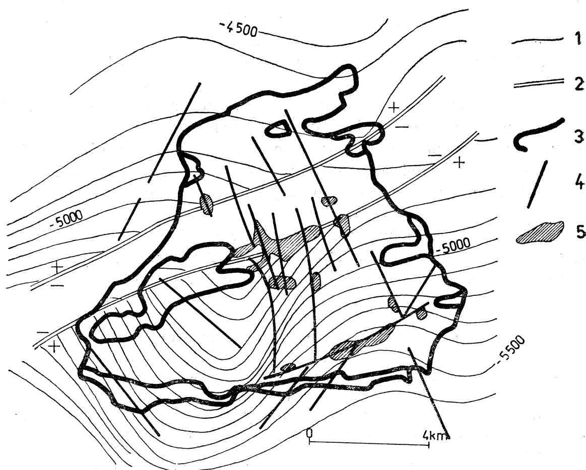
Fig. 9. Mapa strukturalna stropu mezozoiczno-paleozoicznego podłoża fliszu w rejonie okna tektonicznego Mszany Dolnej (według Barczucha et al. , 1981 — nieco zmieniona) z naniesionym położeniem granic na powierzchni terenu jednostek tektonicznych i głównych stref uskokowych. 1 — poziomice strukturalne stropu mezozoiczno-paleozoicznego podłoża fliszu, 2 — uskoki w tym podłożu, 3 — linie nasunięć jednostek tektonicznych na powierzchni terenu, 4 — główne strefy uskokowe na powierzchni terenu, 5 — obszary nagromadzenia wystąpień martwic wapiennych
