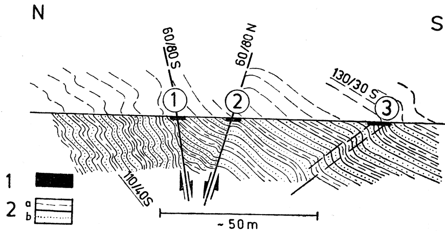
Fig. 7. Schematyczny przekrój geologiczny wzdłuż rzeki Raby z zaznaczonymi odsłonięciami martwic w postaci zlepów (odsl. 1 i 2) oraz pól (odsl. 3) na uskokach opierających i załadowaniach związanych z dużym uskokiem południkowym (patrz Fig. 4). 1 — strefy występowania martwic, 2 — warstwy łupków (a) i piaskowców (b). Na przekroju podano biegi i upady warstw i powierzchni uskokowych oraz przy uskokach strzałkami zaznaczono zwrot ruchu uskokowego
