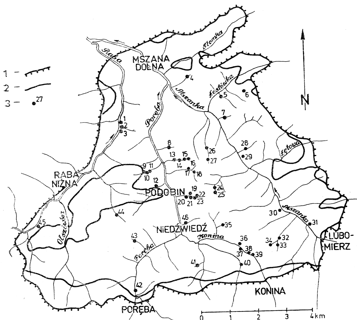
Fig. 2. Lokalizacja wystąpień martwic wapiennych w oknie tektonicznym Mszany Dolnej. 1 — granica nasunięcia jednostki magurskiej, 2 — granica nasunięcia jednostki grybowskiej, 3 — wystąpienia martwic
