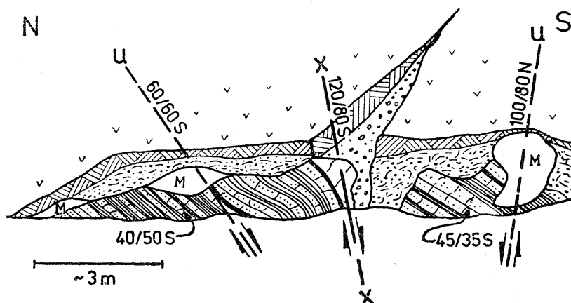
Fig. 6. Rysunek odsłonięcia z martwicami w postaci zlepiów (M) na uskokach niższego rzędu (u) towarzyszących uskocowi głównemu (x-x). Odsłonięcie nr 37 w potoku Konina (lokalizacja na Fig. 2 i 4)
