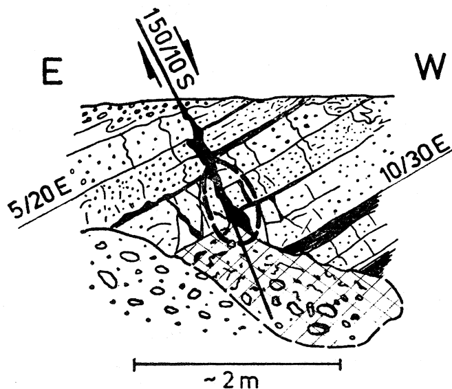
Fig. 8. Rysunek niewielkiego uskoku ze źródłem szczelinowym i polewą wapienną (obszar zakratkowany) poniżej strefy wypływu (obszar obwiedzony linią przerywaną) tego źródła. Strzałkami zaznaczono zwrot ruchu uskokowego. Lewy orograficznie dopływ potoku Poręba we wsi Podobin. Odsłonięcie nr 19 (lokalizacja na fig. 2 i 4)
