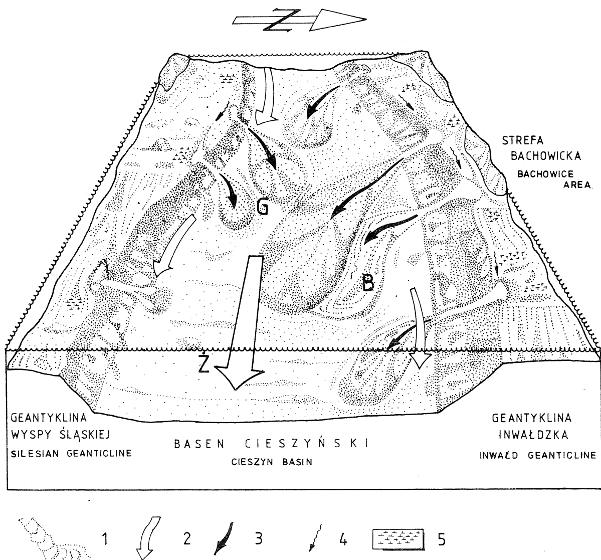
Fig. 21. Paleogeografia basenu cieszyńskiego w tytonie (wg Książkiewicza, 1956, 1960a; Nowaka, 1973; zmienione i uszczegółowione). 1 — spływy gruzowo-mułowe; 2 — prądy denne; 3 — prądy zawieszinowe; 4 — prądy litoralne; 5 — strefy gromadzenia mułu węglanowego; G — rejon Goleiszowa; B — rejon Bielska-Białej; Ż — rejon Żywca (położenie przed kompresją geosynkliny)
