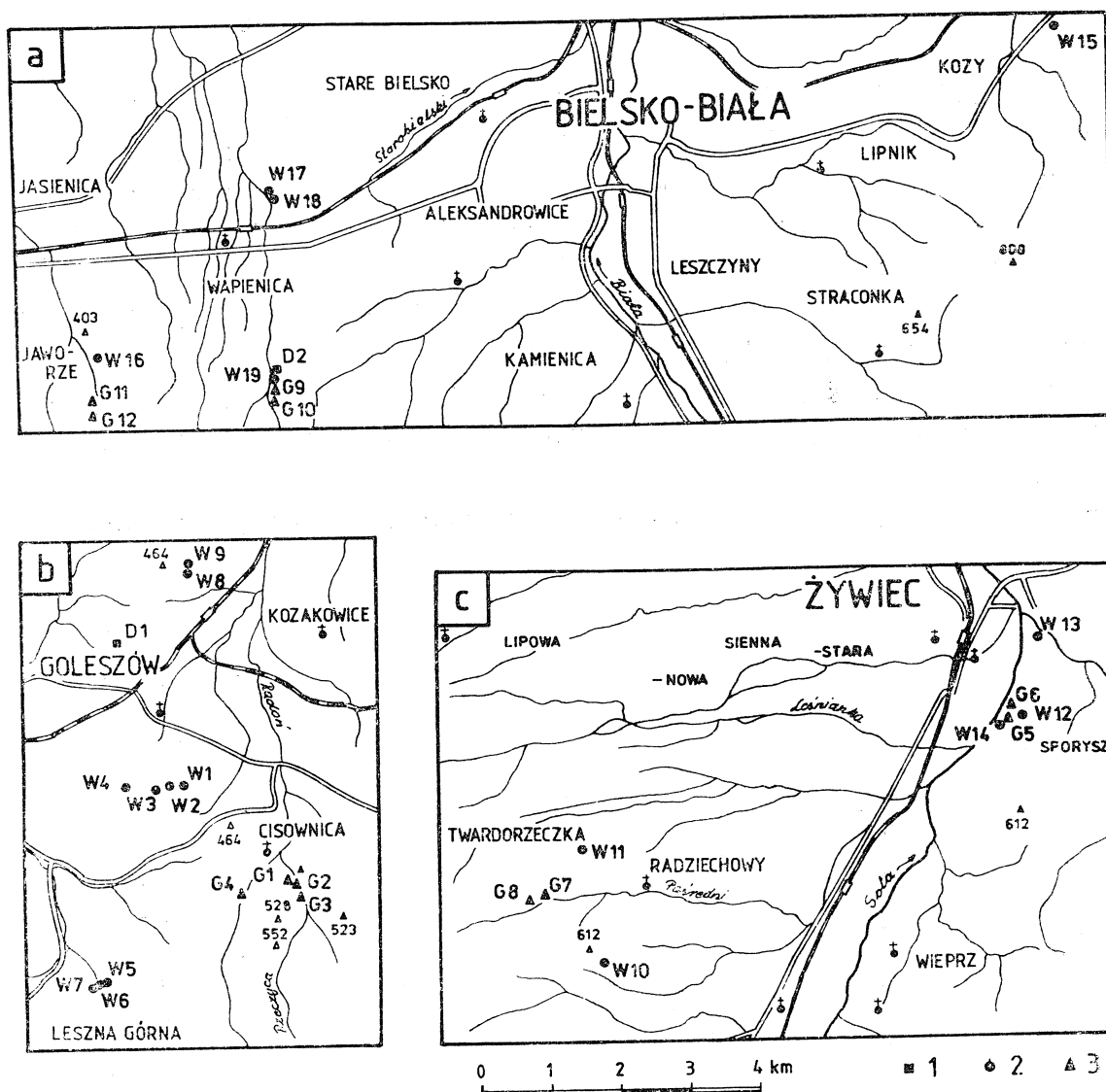
Fig. 4. Lokalizacja profili wytypowanych do badań ilościowych. a — region Bielska-Białej; b — region Goleszowa; c — region Żywca; 1 — łupki cieszyńskie dolne; 2 — wapień cieszyński; 3 — łupki cieszyńskie górne
