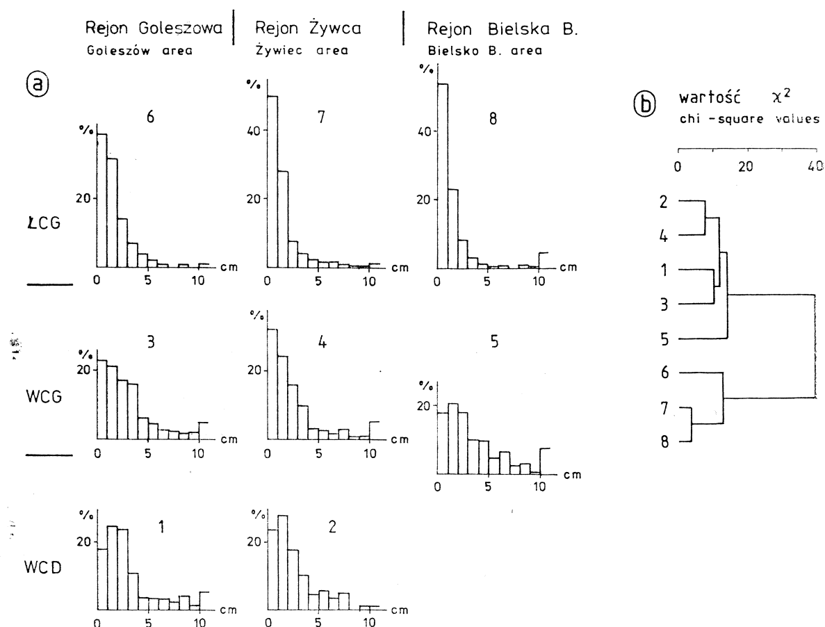
Fig. 5. (a) Rozkłady miąższości warstw psammitów z laminacją równoległą. (b) Porównanie rozkładów za pomocą testu \chi^2 . WCD — wapienie cieszyńskie dolne; WCG — wapienie cieszyńskie górne; LCG — łupki cieszyńskie górne
