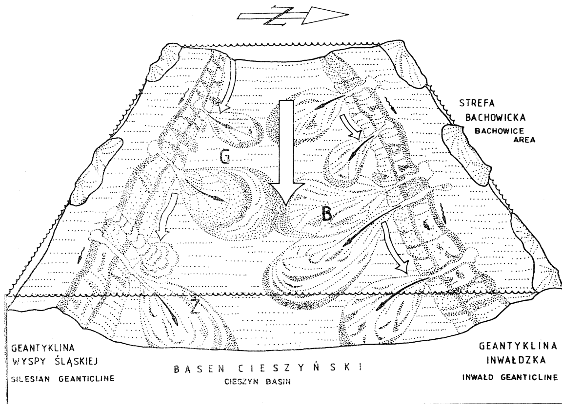
Fig. 23. Paleogeografia basenu cieszyńskiego w walanżynie. Objaśnienia jak na figurze 21
