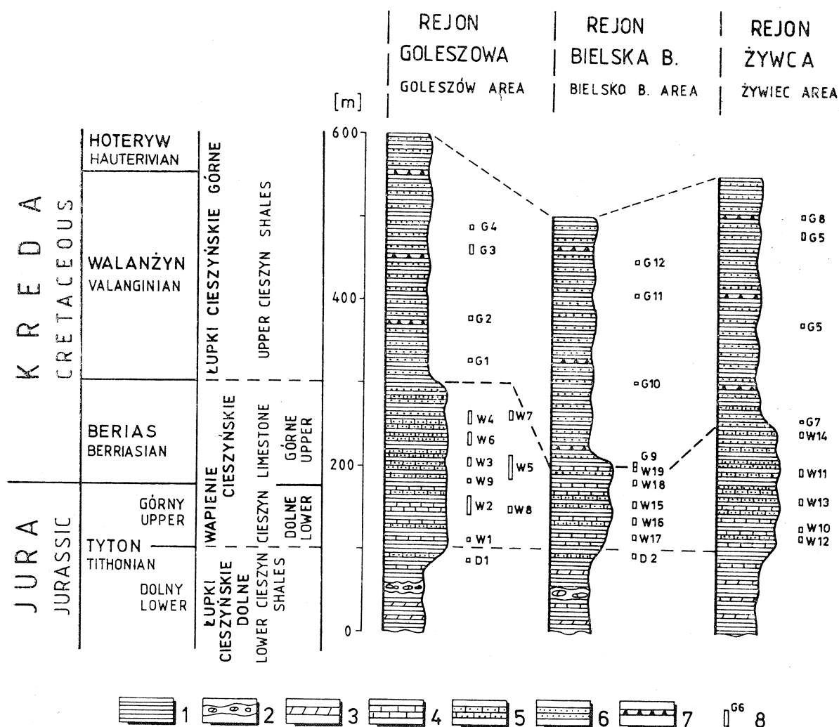
Fig. 3. Lokalizacja stratygraficzna profili wytypowanych do badań ilościowych w syntetycznym profilu warstw cieszyńskich. 1 — łupki margliste; 2 — żwirowce ilaste; 3 — margle; 4 — wapienie pelityczne; 5 — wapienie detrytyczne; 6 — piaskowce; 7 — syderyty; 8 — zbadane profile
