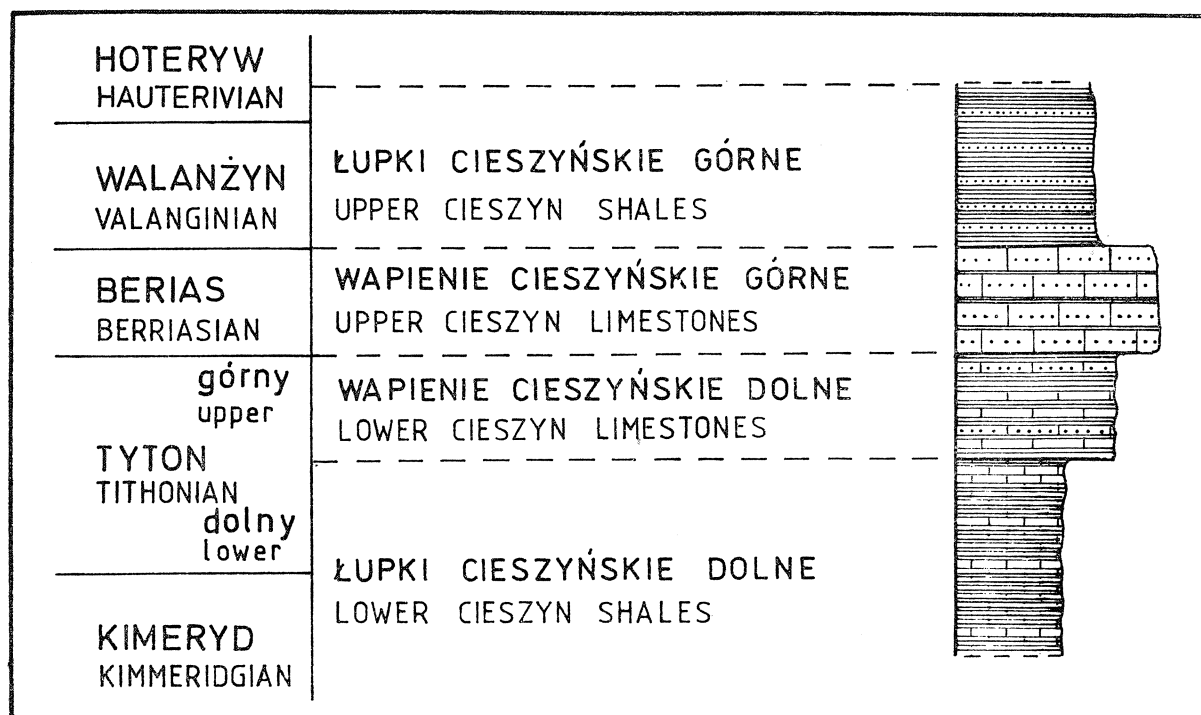
Fig. 2. Schemat litostratygraficzny warstw cieszyńskich (wg Nowaka, 1973; Koszarskiego & Ślączi, 1973; uproszczone)
