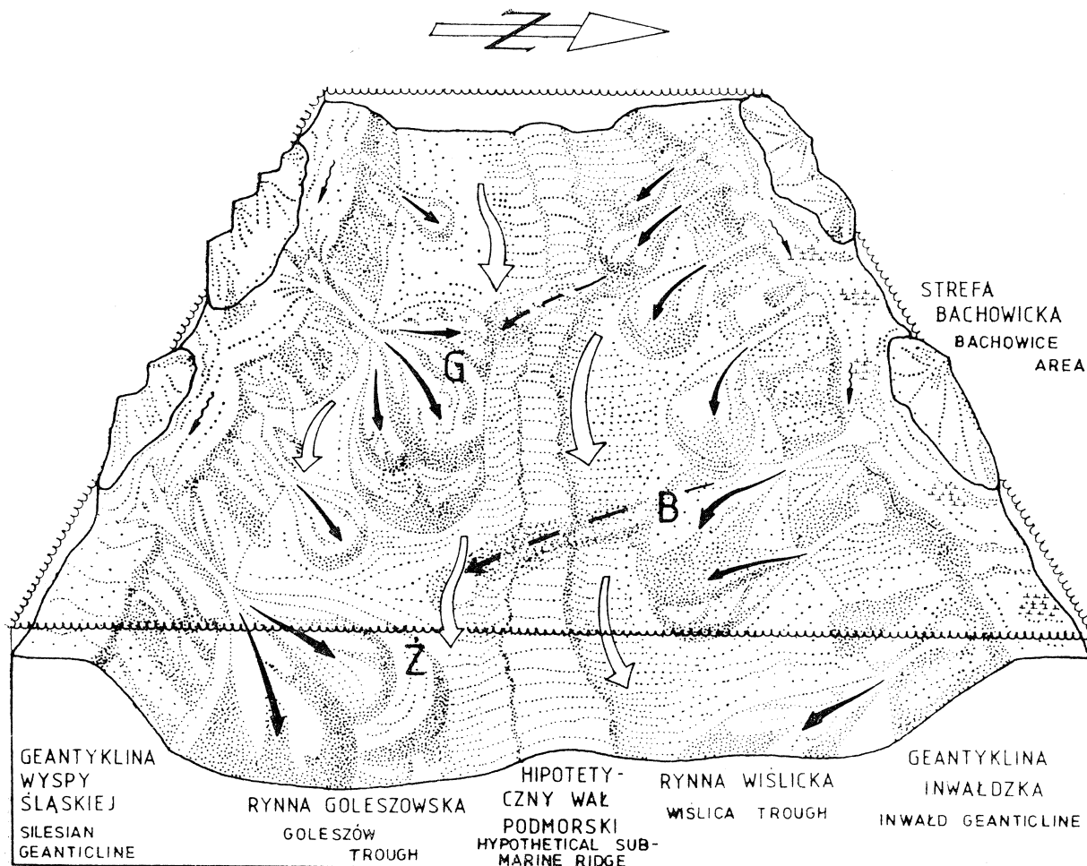
Fig. 22. Paleogeografia basenu cieszyńskiego w beriasie. Objasnienia jak na figurze 21
