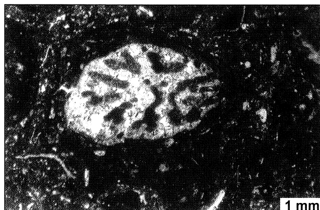
Fig. 13. Floatstone – wackestone with scleractinian coral (fragment of colony? pers. commun. E. Morycowa, B. Kołodziej, 2001); Księża Hill
