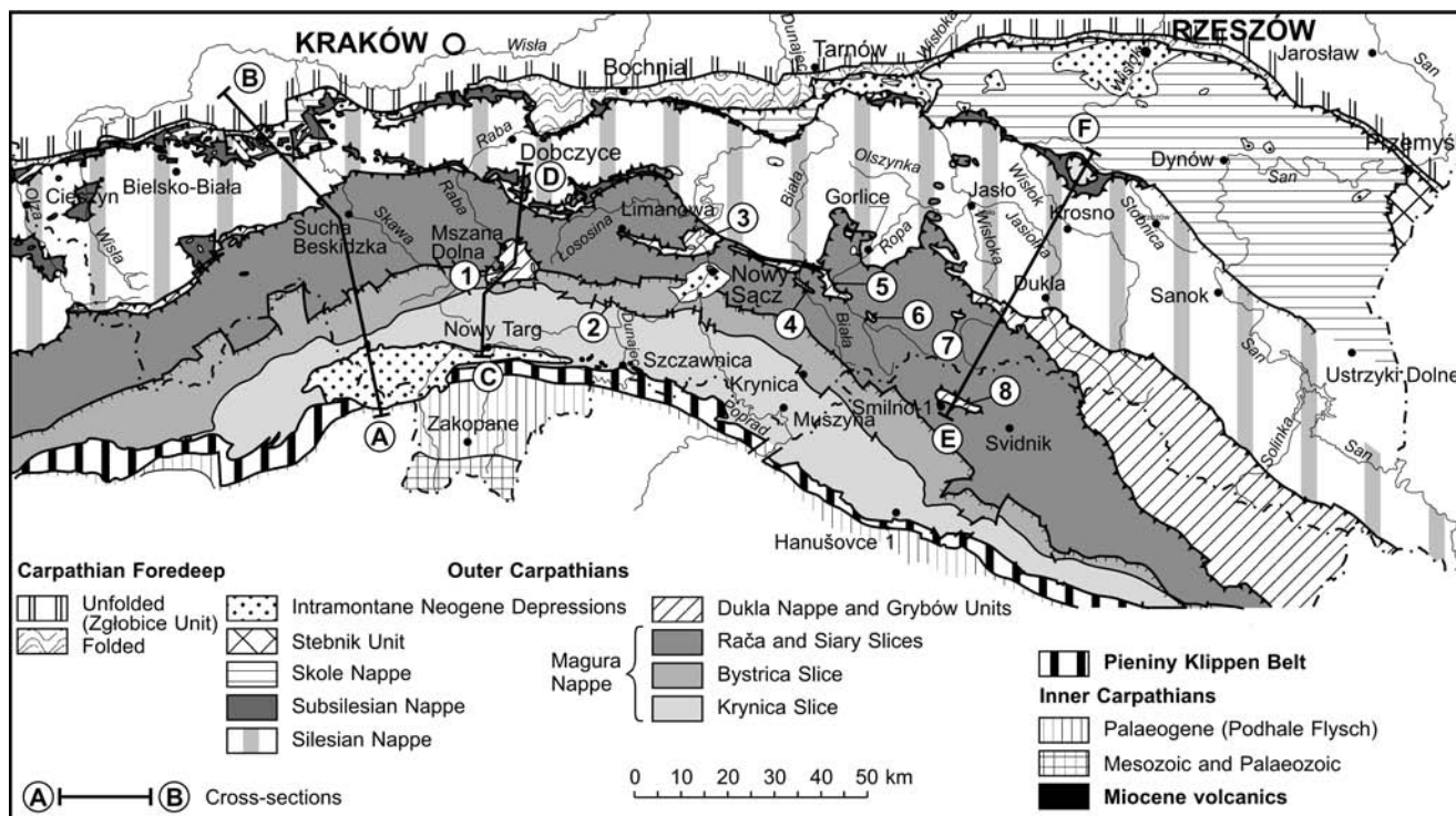
Fig. 1. Tectonic sketch of the Outer West Carpathians (based on Żytko et al., 1989 ; simplified). Tectonic windows: 1 – Mszana Dolna, 2 – Szczawa, 3 – Klęczany–Pisarzowa, 4 – Grybów, 5 – Ropa, 6 – Ucie Gorlickie, 7 – Gwiłtkowa, 8 – Smilno
